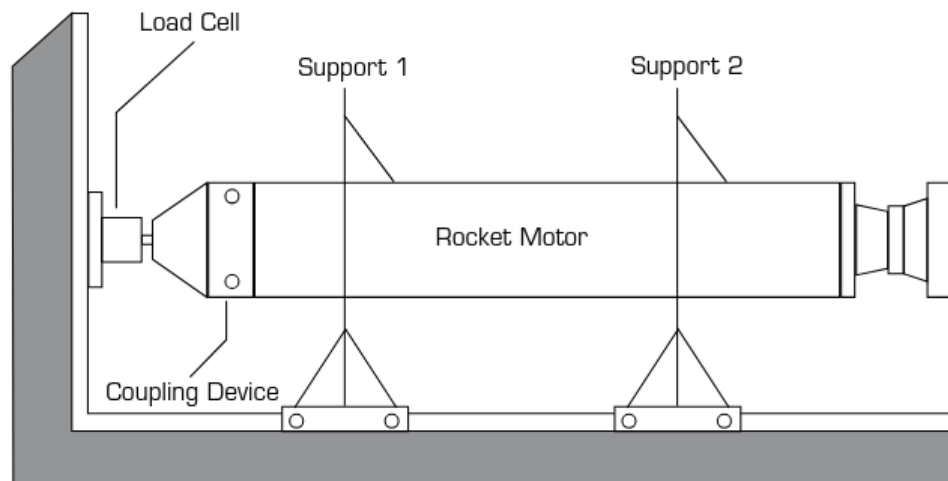
Slika 1: Shema tipičnega statičnega testa [5]
