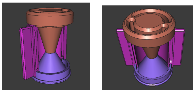
Slika 6: Načrt modelčka za vlivanje šob
