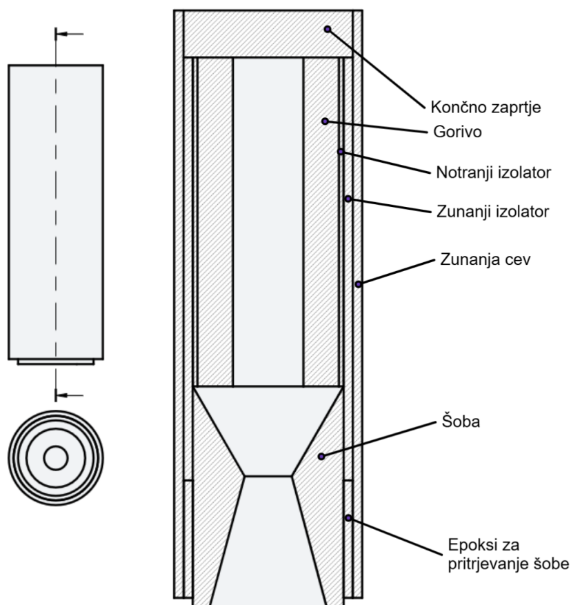
Slika 7: Shema motorja
