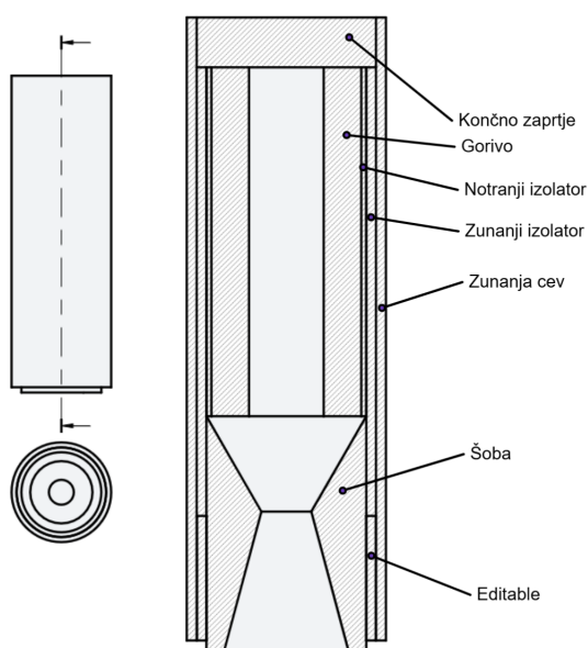
Slika 5: Shema motorja
