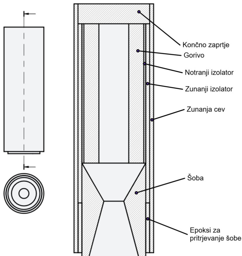
Slika 5: Shema motorja
