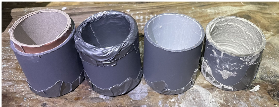
Slika 1: Prvi test: karton, tekstilni lepilni trak, kontrola, cement
