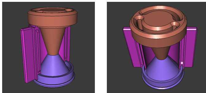
Slika 5: Načrt modelčka za ulivanje šob
