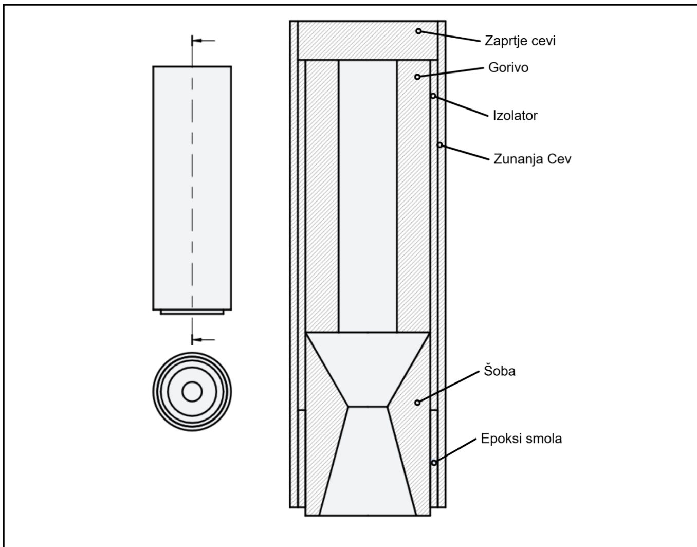
Slika 5: Shema motorja
