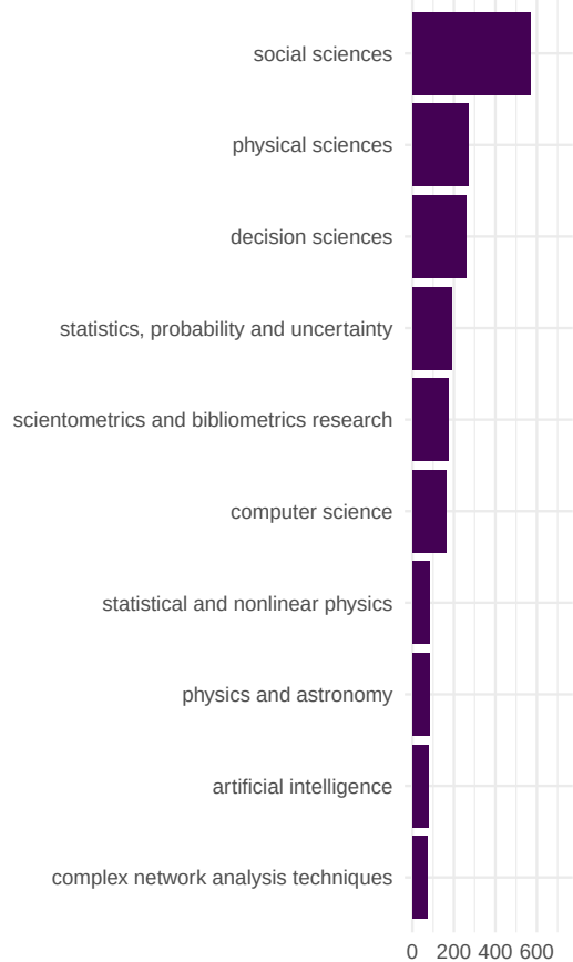
J. Informetrics
