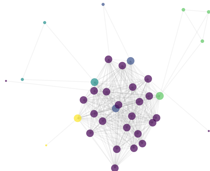
DrL
