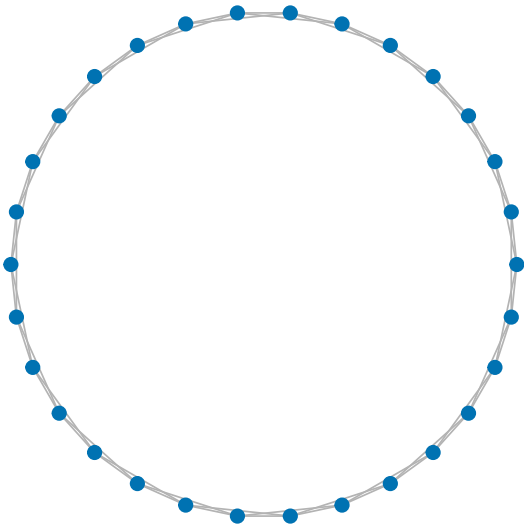
Ring Lattice (k=4)
