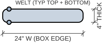
CUSHION SECTION — BOX EDGE
