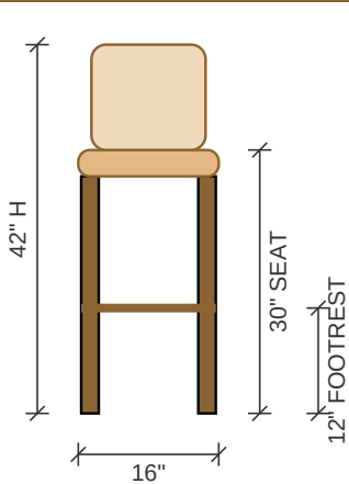
BAR STOOL — FRONT
