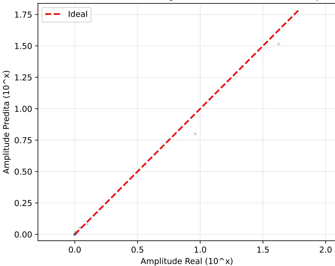
Real vs Predito (escala original) - 40 amostras de validação
