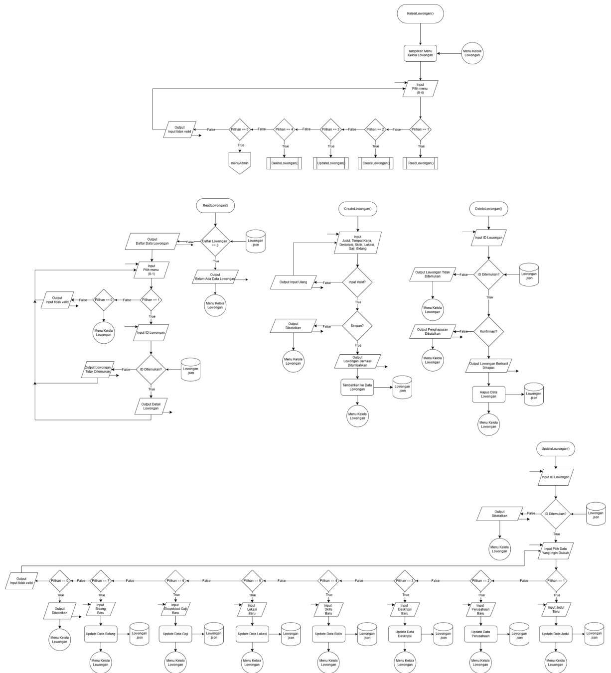
Gambar 2.6 Flowchart Menu Kelola Lowongan (Admin)
