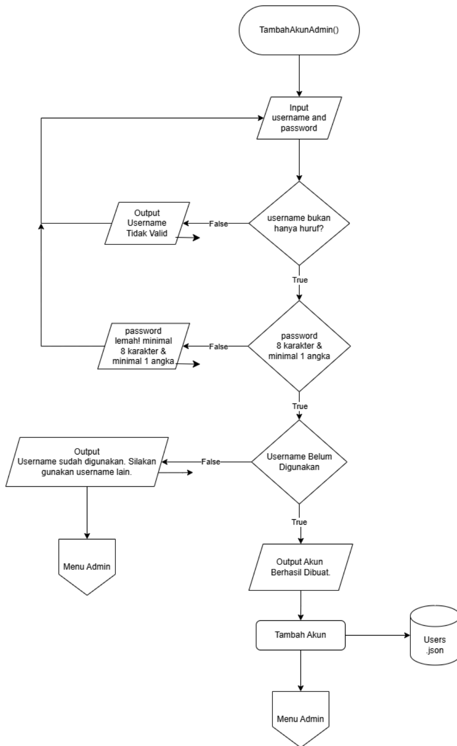
Gambar 2.8 Flowchart Fitur Tambah Akun Admin baru (Admin)
