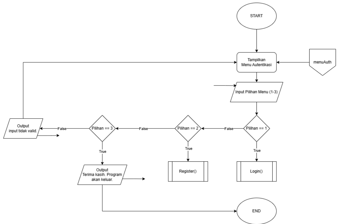
Gambar 2.1 Flowchart Alur Utama
