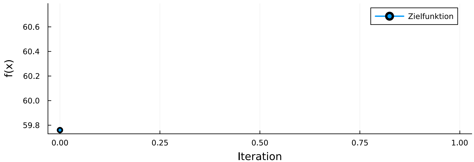
P2: Quadratisches Problem mit Gleichheitsnebenbedingungen
