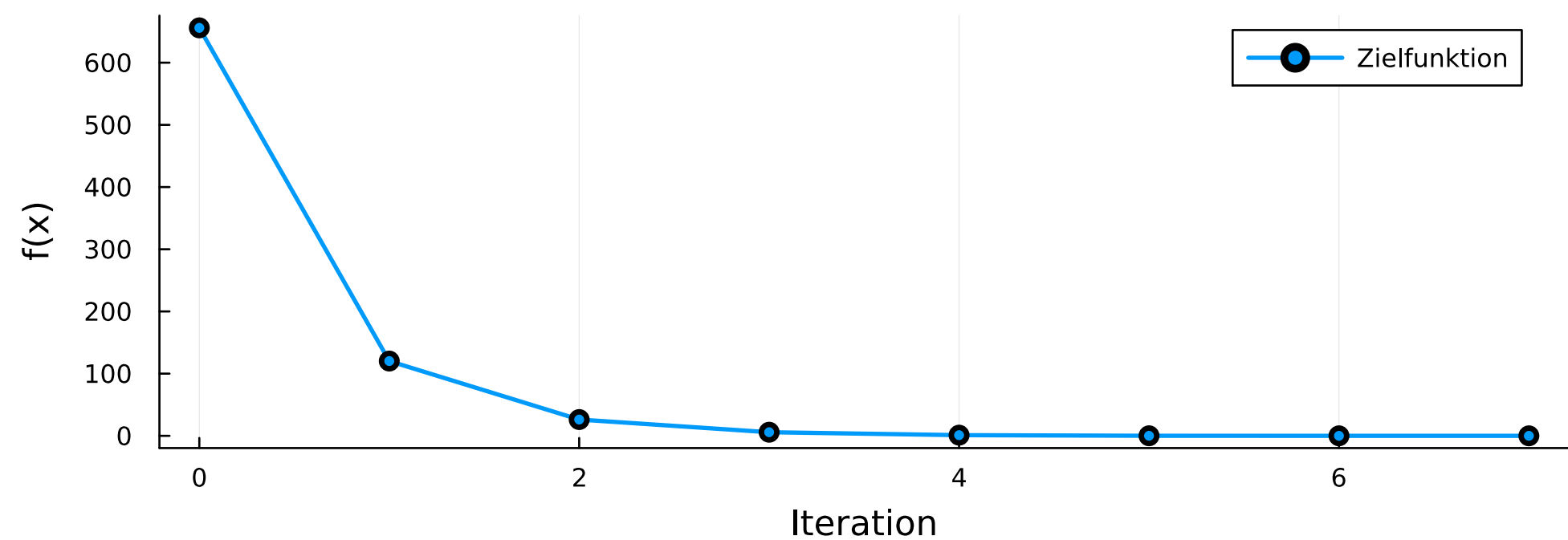
P3: Nichtlineares Problem mit Gleichheitsnebenbedingung
