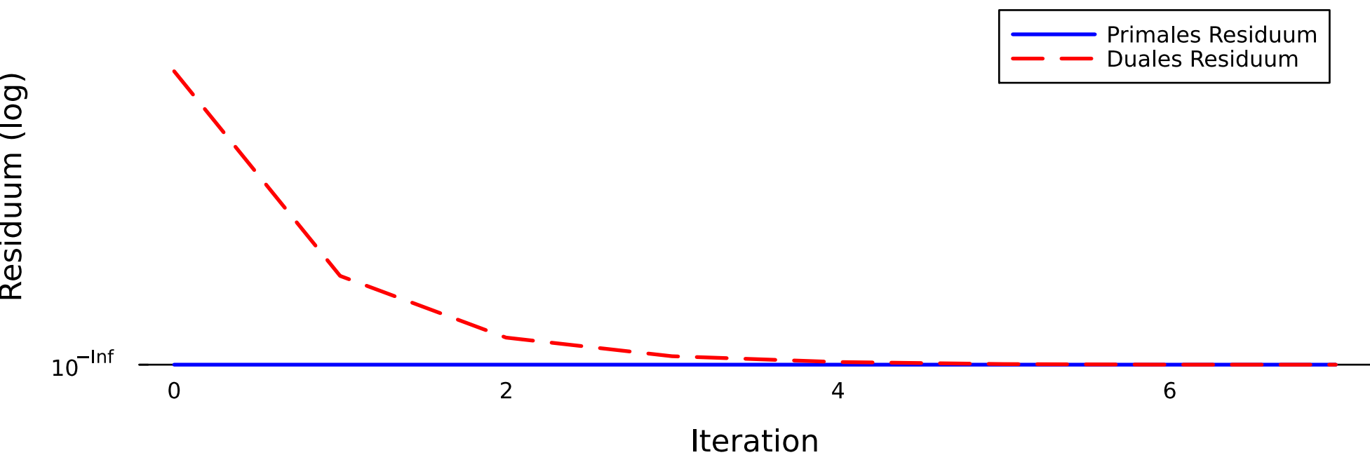
P3: Nichtlineares Problem mit Gleichheitsnebenbedingung
