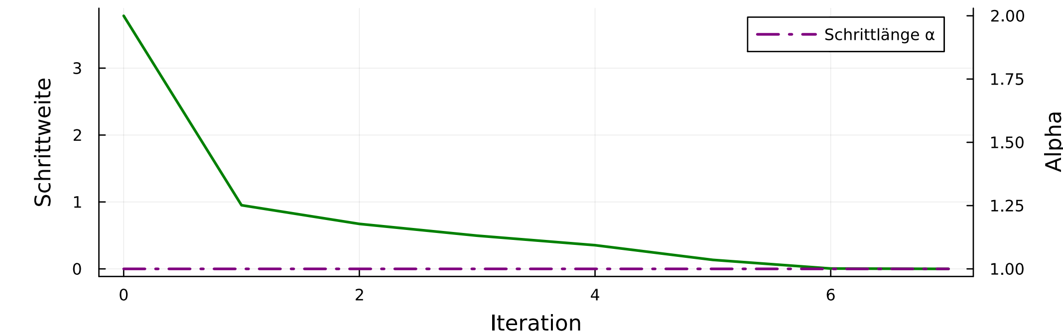
P3: Nichtlineares Problem mit Gleichheitsnebenbedingung
