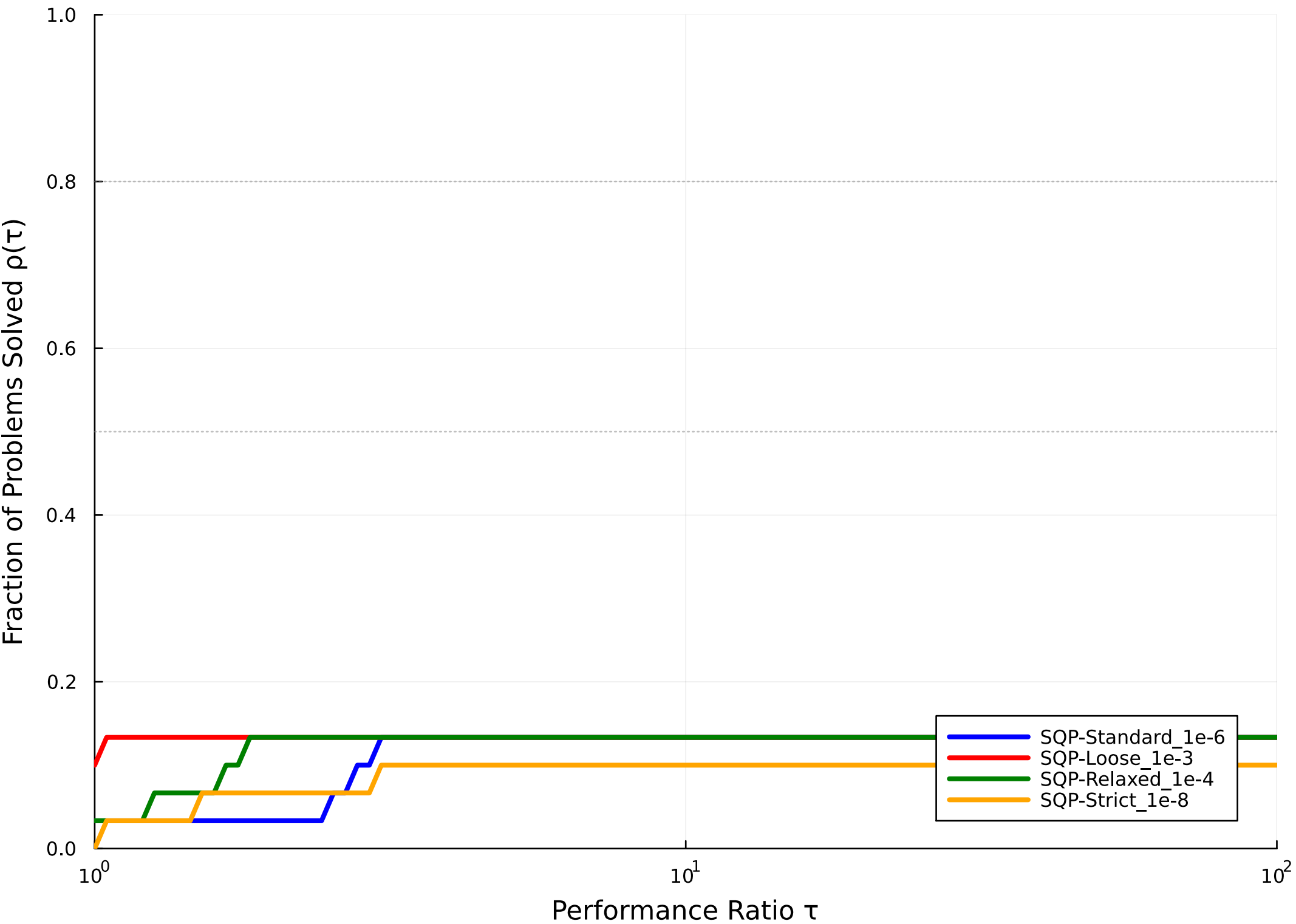
Performance Profile: tolerance_comparison (Funktionsauswertungen)
