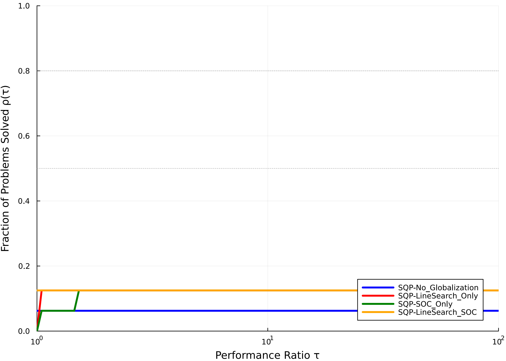
Performance Profile: globalization_strategies (Funktionsauswertungen)
