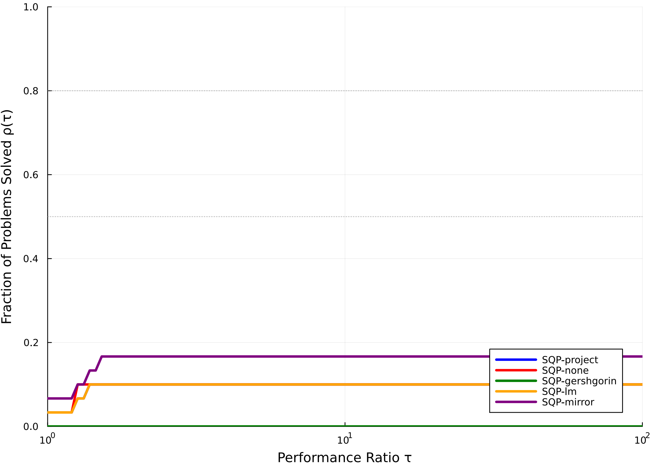
Performance Profile: hessian_convexification (Funktionsauswertungen)
