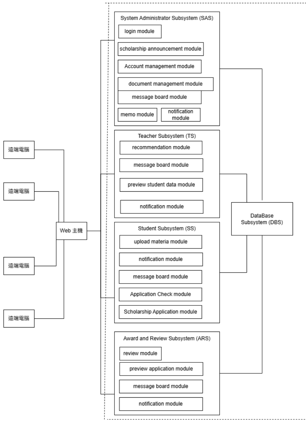
圖一 NUKSAS的系統架構
