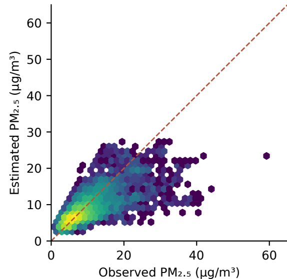
HGB
