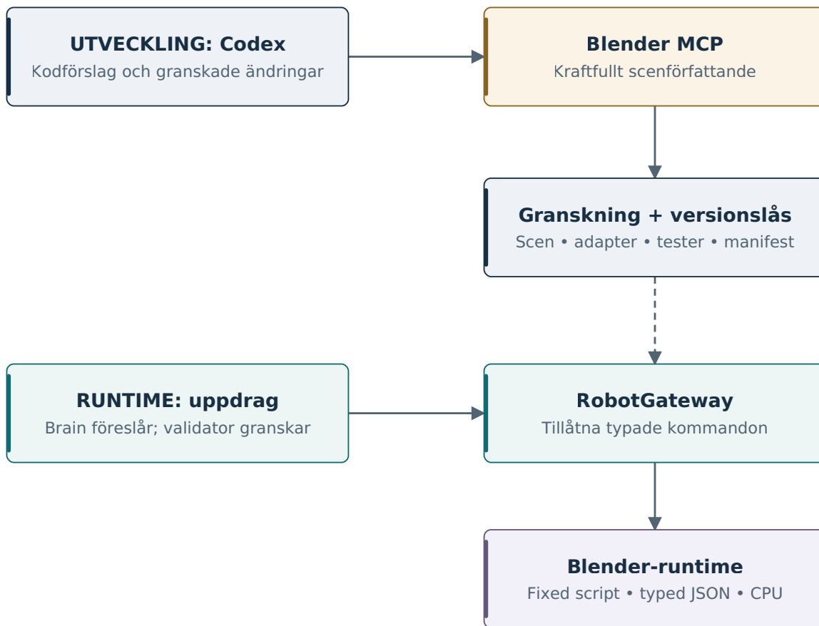
Figur 6. Egen behörighetsmodell. Codex och MCP kan hjälpa till med scenförfattande i en isolerad utvecklingsmiljö. Granskade och versionshanterade artefakter förs sedan till körmiljön. RobotGateway accepterar enbart det avgränsade runtime-kontraktet.
