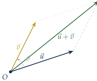
Figure 5.1: Addition de vecteurs et angle formé.
