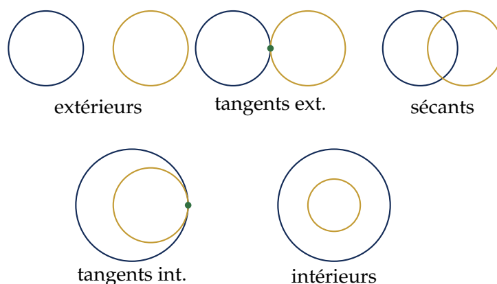
Figure 6.3: Cinq positions relatives de deux cercles.
