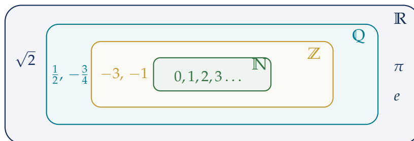
Figure 3.1: Hiérarchie des ensembles de nombres : \mathbb{N} \subset \mathbb{Z} \subset \mathbb{Q} \subset \mathbb{R} . Chaque ensemble contient le précédent, plus de nouveaux nombres.
