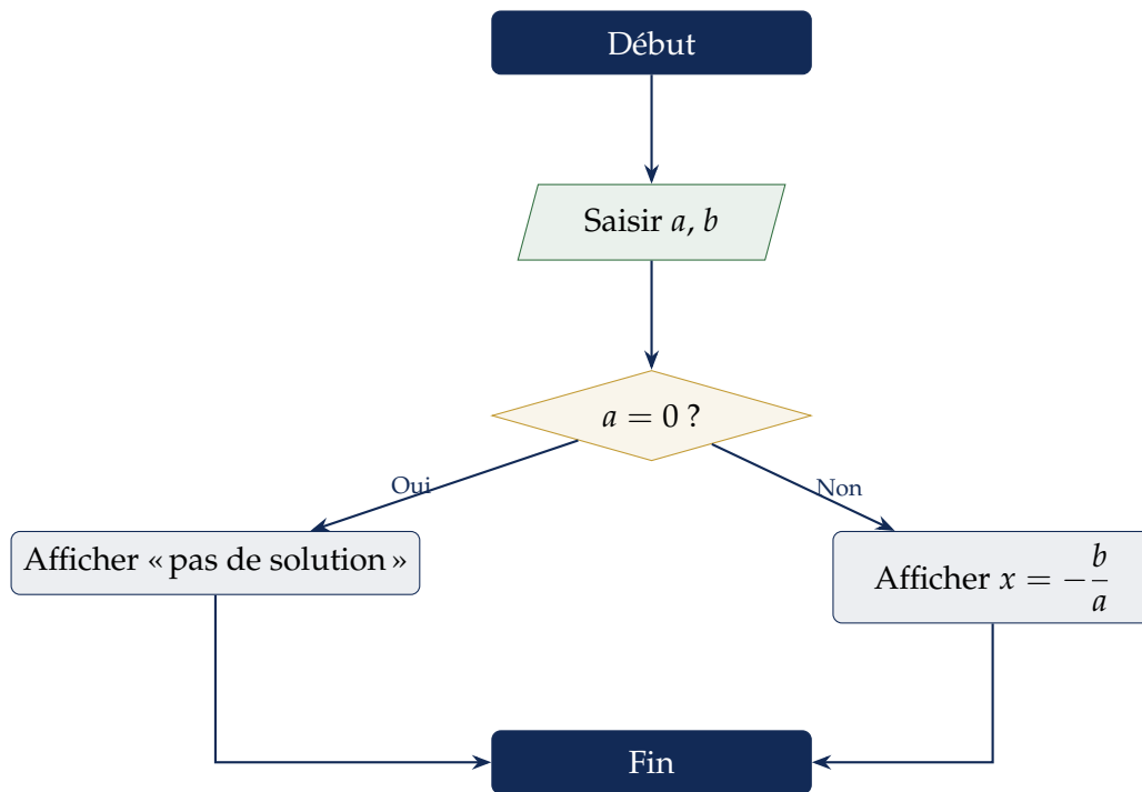
Figure 2.2: Organigramme : résolution de ax + b = 0 .
