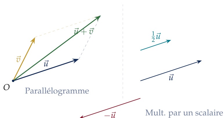
Figure 5.3: Gauche : addition de vecteurs (règle du parallélogramme). Droite : multiplication de \vec{u} par un scalaire : \frac{1}{2}\vec{u} (demi-vecteur, bleu) ; -\vec{u} (opposé, rouge).
