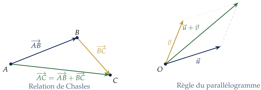
Figure 5.2: Addition de vecteurs : relation de Chasles (gauche) et règle du parallélogramme (droite).
