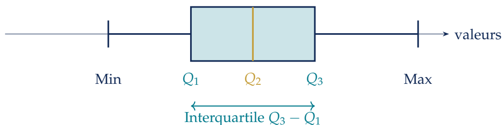
Figure 9.2: Boîte à moustaches : cinq indicateurs.
