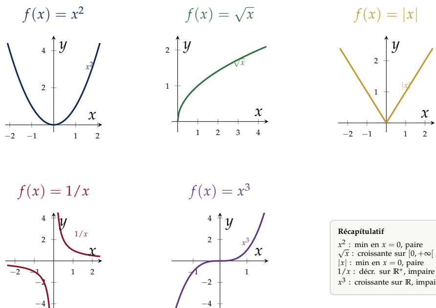
Figure 7.2: Les cinq fonctions de référence — chacune avec son domaine et ses propriétés.
