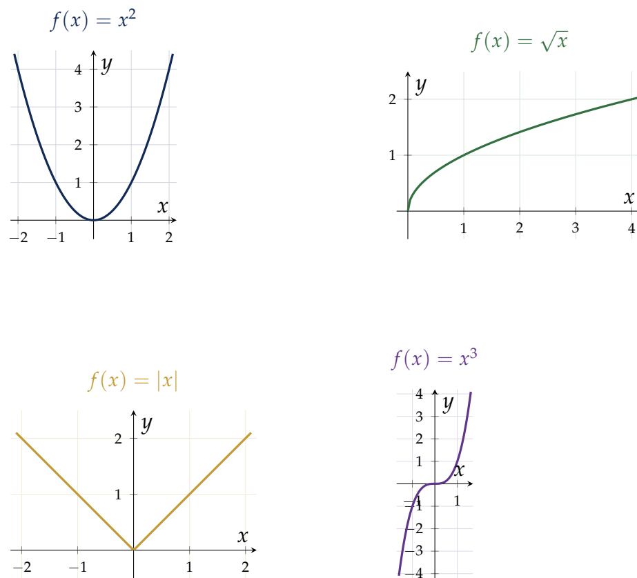
Figure 7.1: Fonctions de référence au programme : graduations régulières et identiques sur chaque axe.
