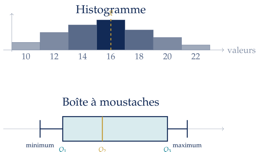
Figure 9.3: Lire une distribution : l'histogramme montre la forme générale ; la boîte à moustaches résume les 5 indicateurs essentiels. Ici la distribution est légèrement asymétrique : la médiane Q_2 (orange) est à gauche de la moyenne \bar{x} (orange, tireté dans l'histogramme).
