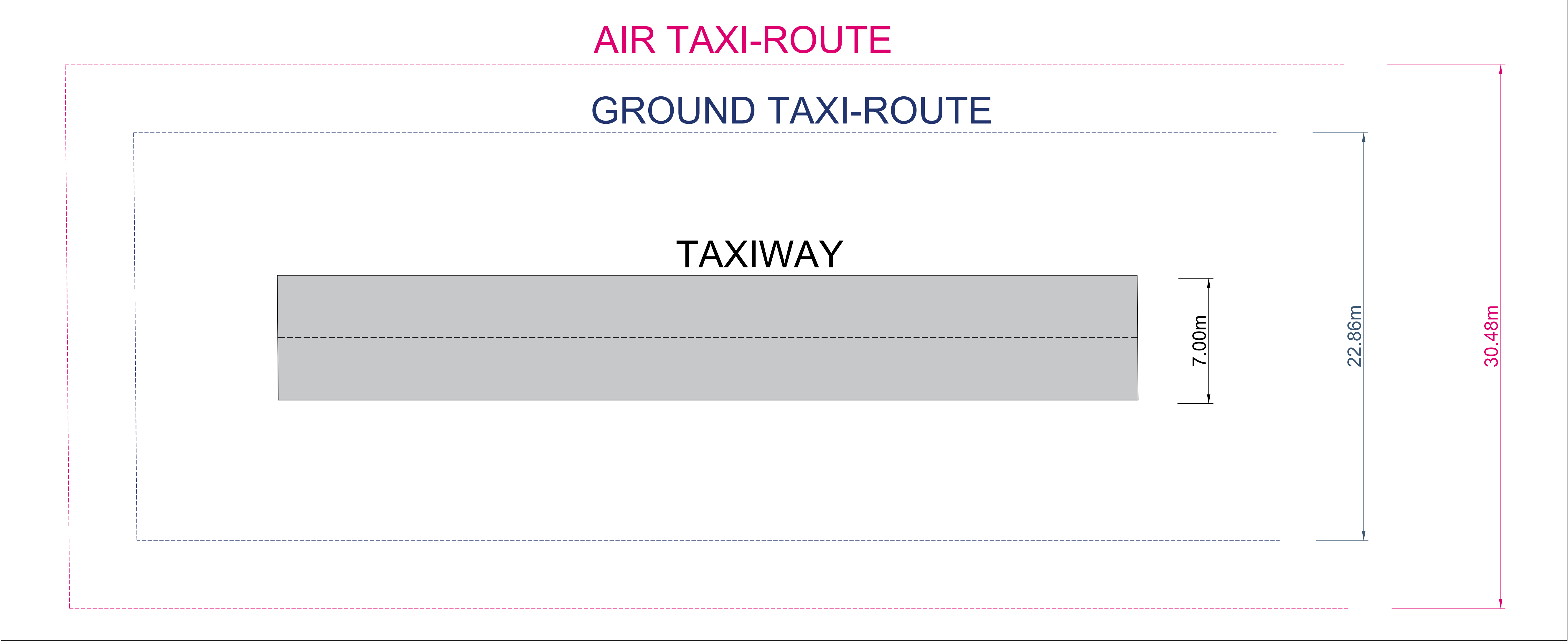
PISTA E ROTA DE TÁXI TERRESTRE E AÉREO - PLANTA ESCALA 1:125
