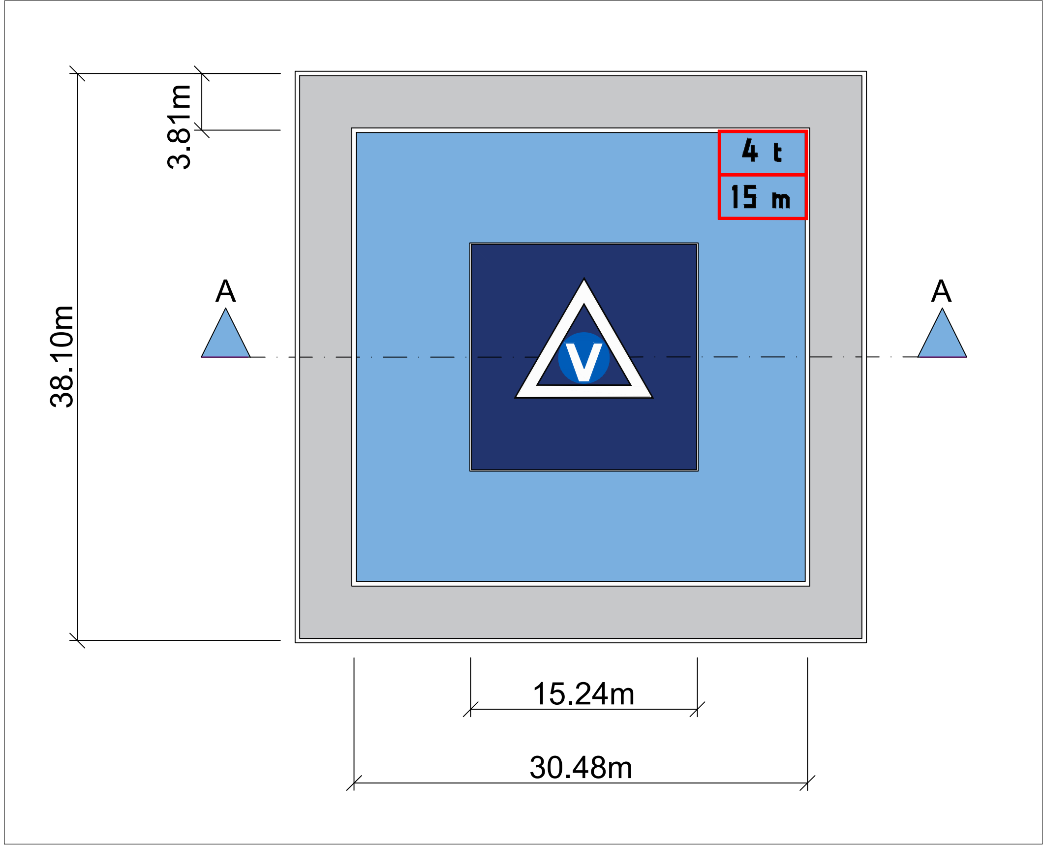
FATO E ÁREA DE SEGURANÇA ASSOCIADA - PLANTA ESCALA 1:250
