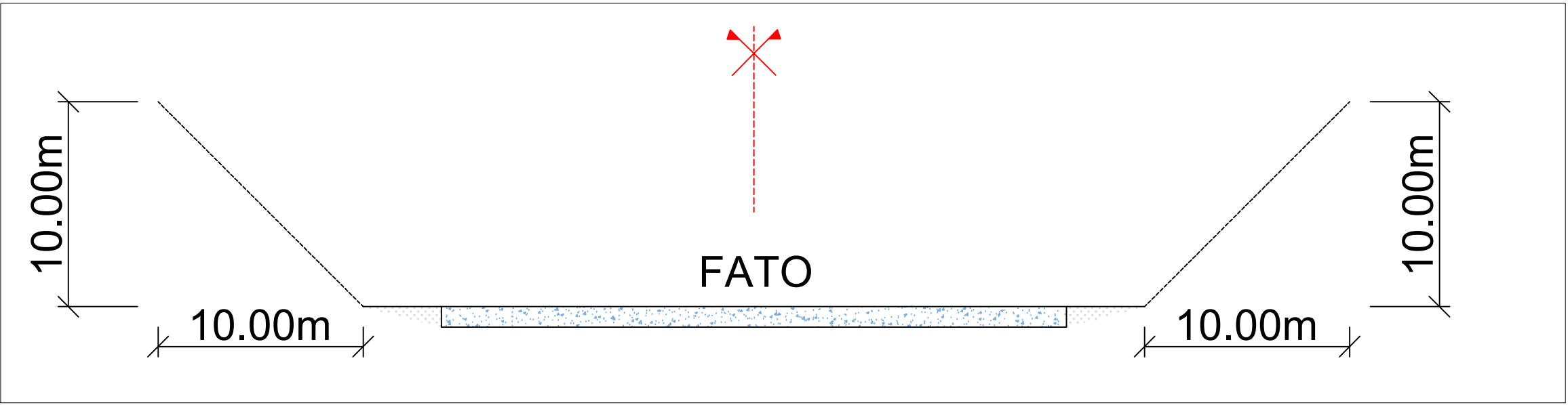
RAMPA LATERAL PROTEGIDA - CORTE AA ESCALA 1:250
