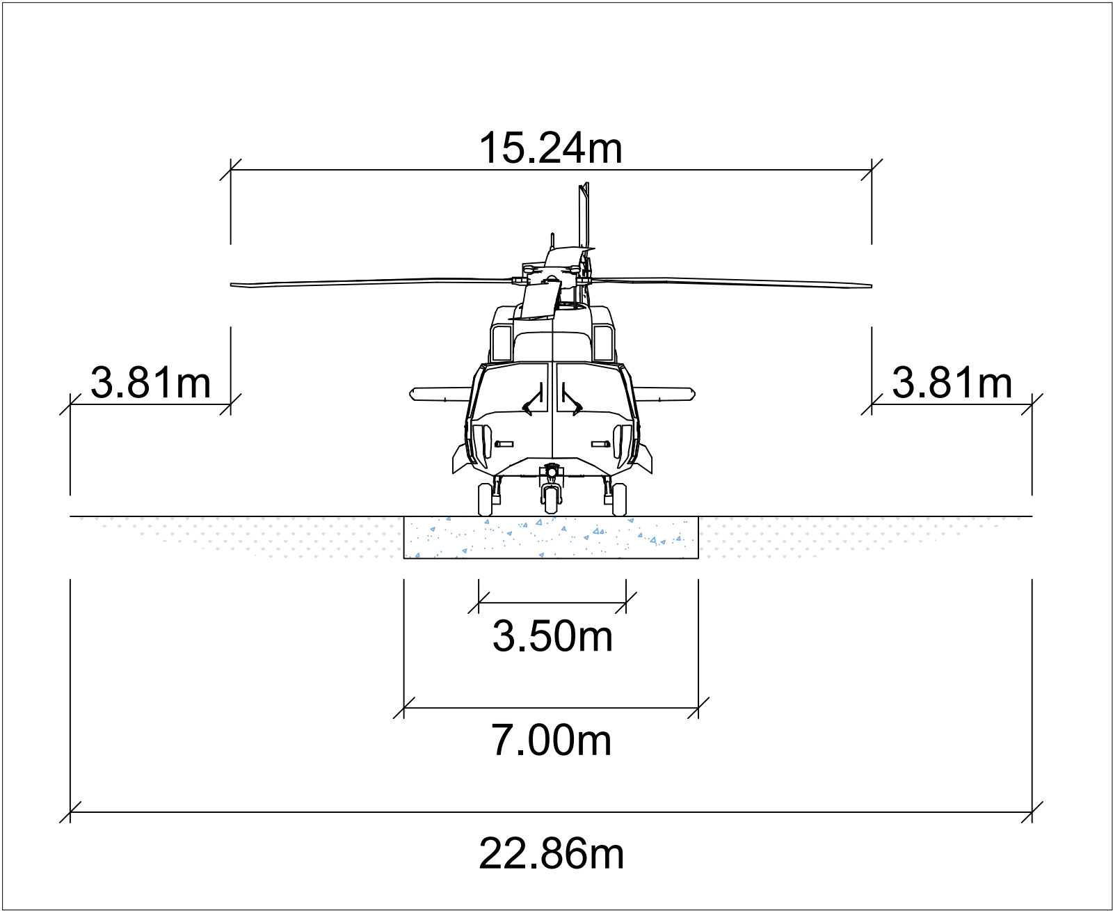
PISTA E ROTA DE TÁXI TERRESTRE - VISTA ESCALA 1:125
