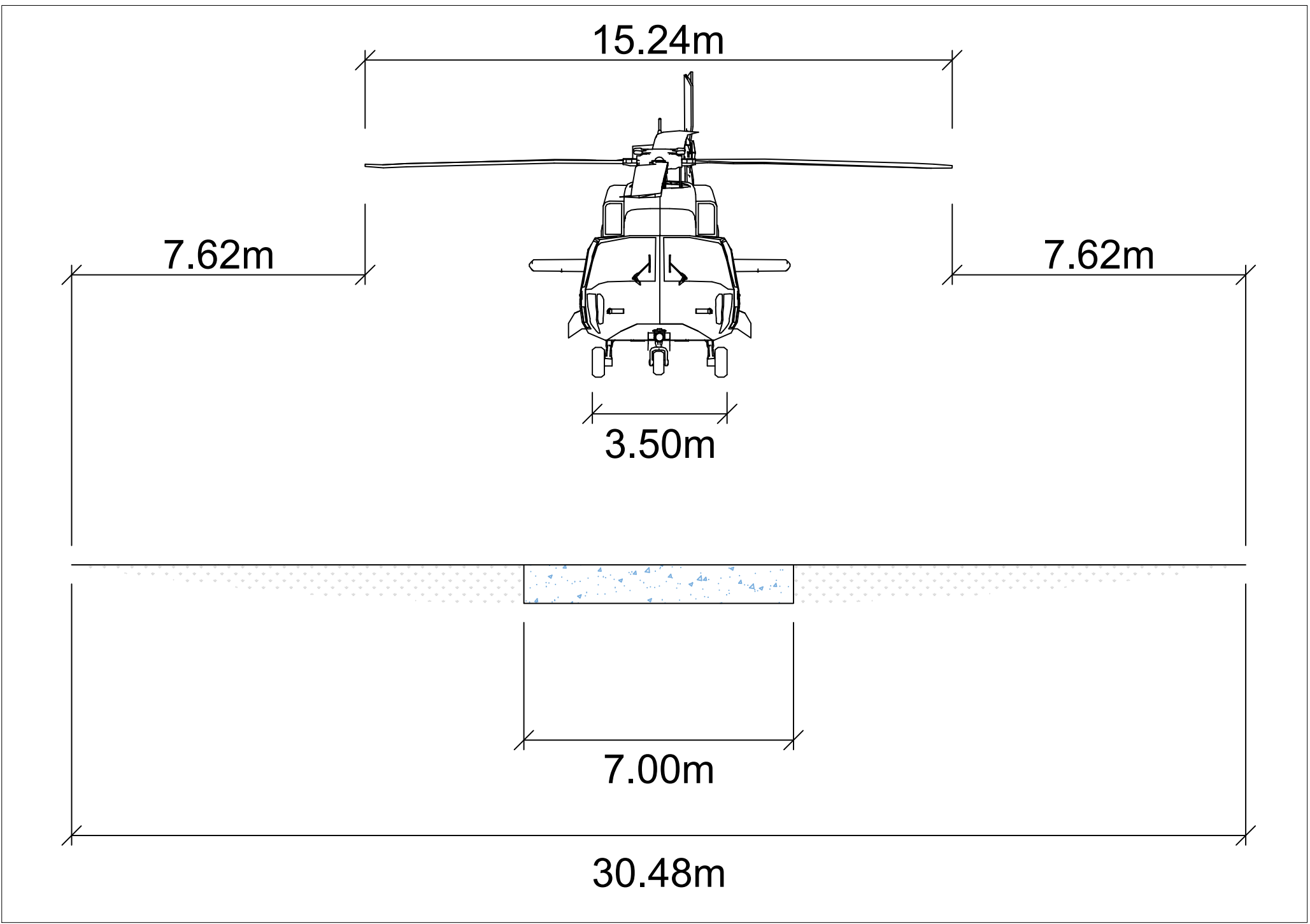
PISTA E ROTA DE TÁXI AÉREO - VISTA ESCALA 1:125
