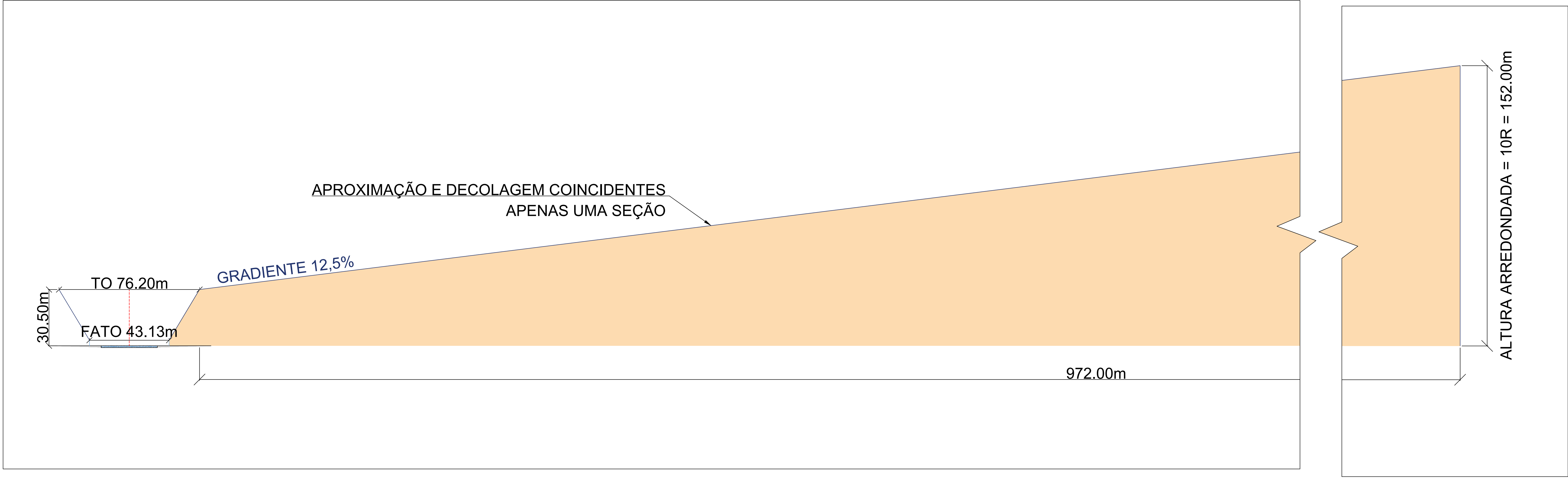
SUPERFÍCIE DE PROTEÇÃO EASA UMA DIREÇÃO - CORTE AA ESCALA 1:1000
