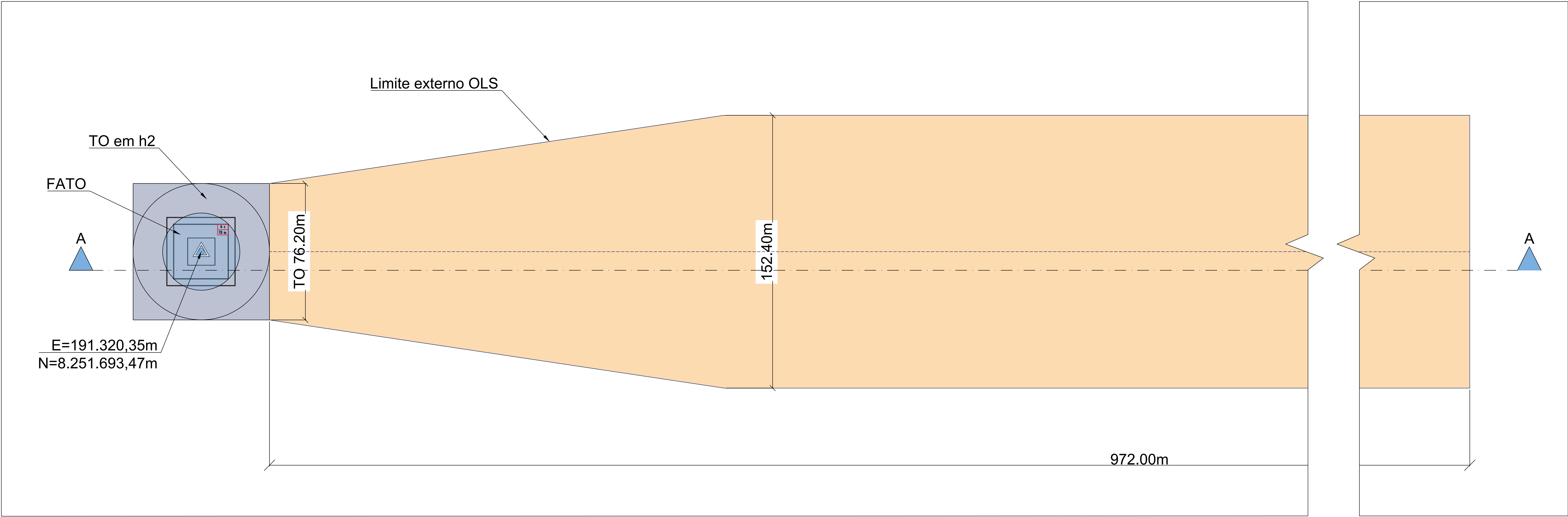
SUPERFÍCIE DE PROTEÇÃO EASA UMA DIREÇÃO - PLANTA ESCALA 1:1000
