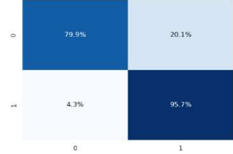
7. FP32 Hata Matrisi (%)
