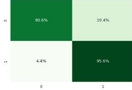
8. INT8 Hata Matrisi (%)
