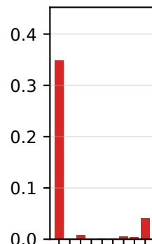
GPT-2 -- FER ↓
