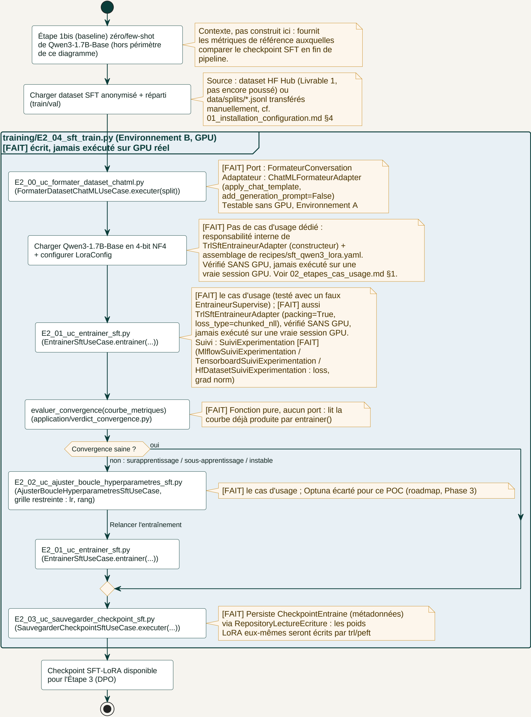
Étape 2 : Pipeline SFT + LoRA Diagramme d'activité : E2_00 à E2_03 et TrlSftEntraîneurAdapter/E2_04_sft_train.py écrits et testés (jamais exécutés sur GPU réel, cf. docs/03_etape2_sft/)
