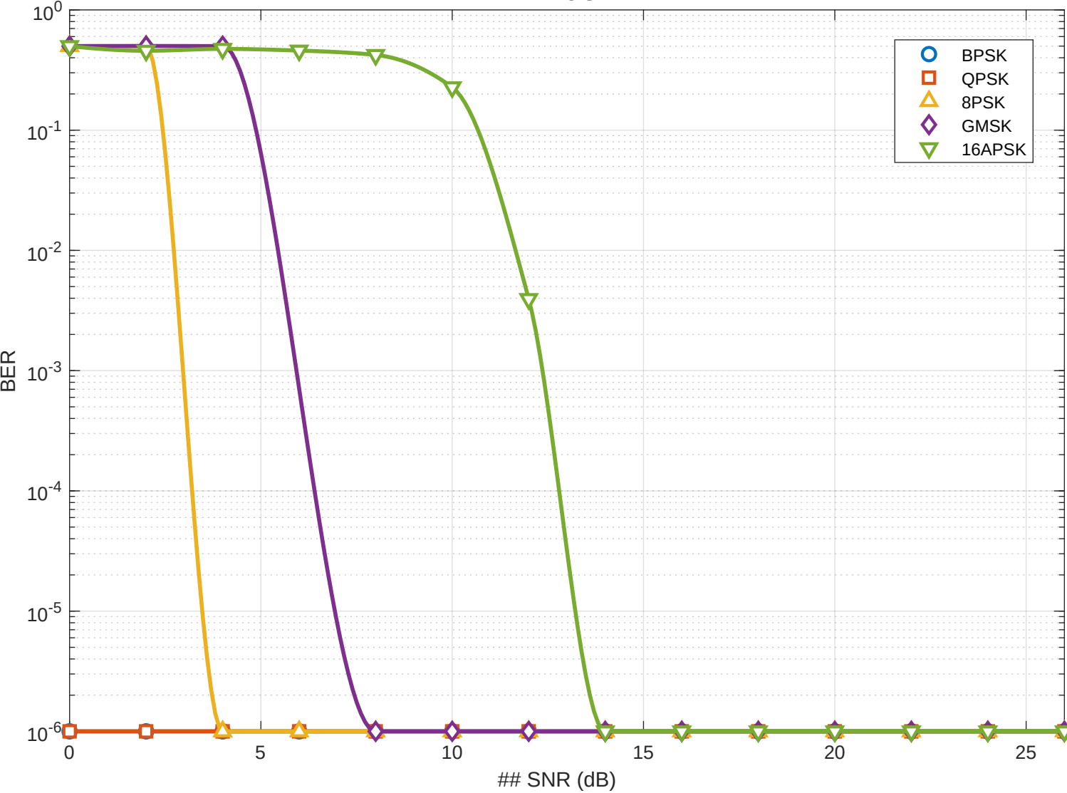
BER vs SNR
