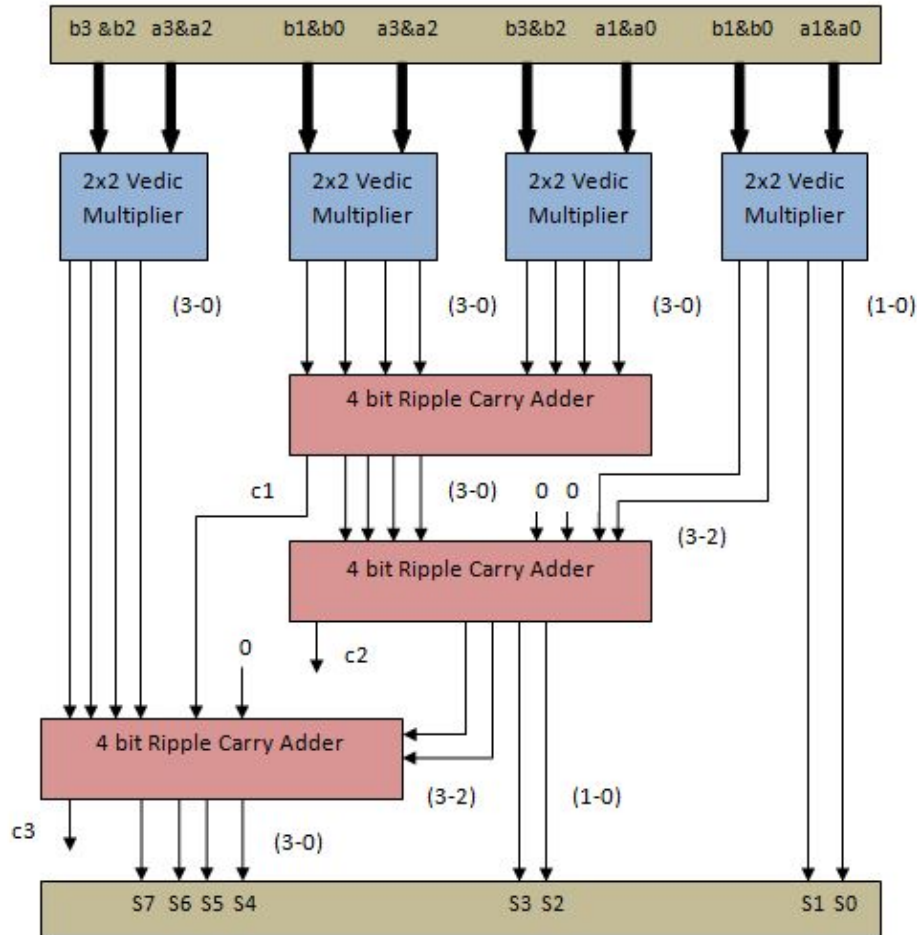
Figure 2.3: 4x4 Vedic Multiplier
