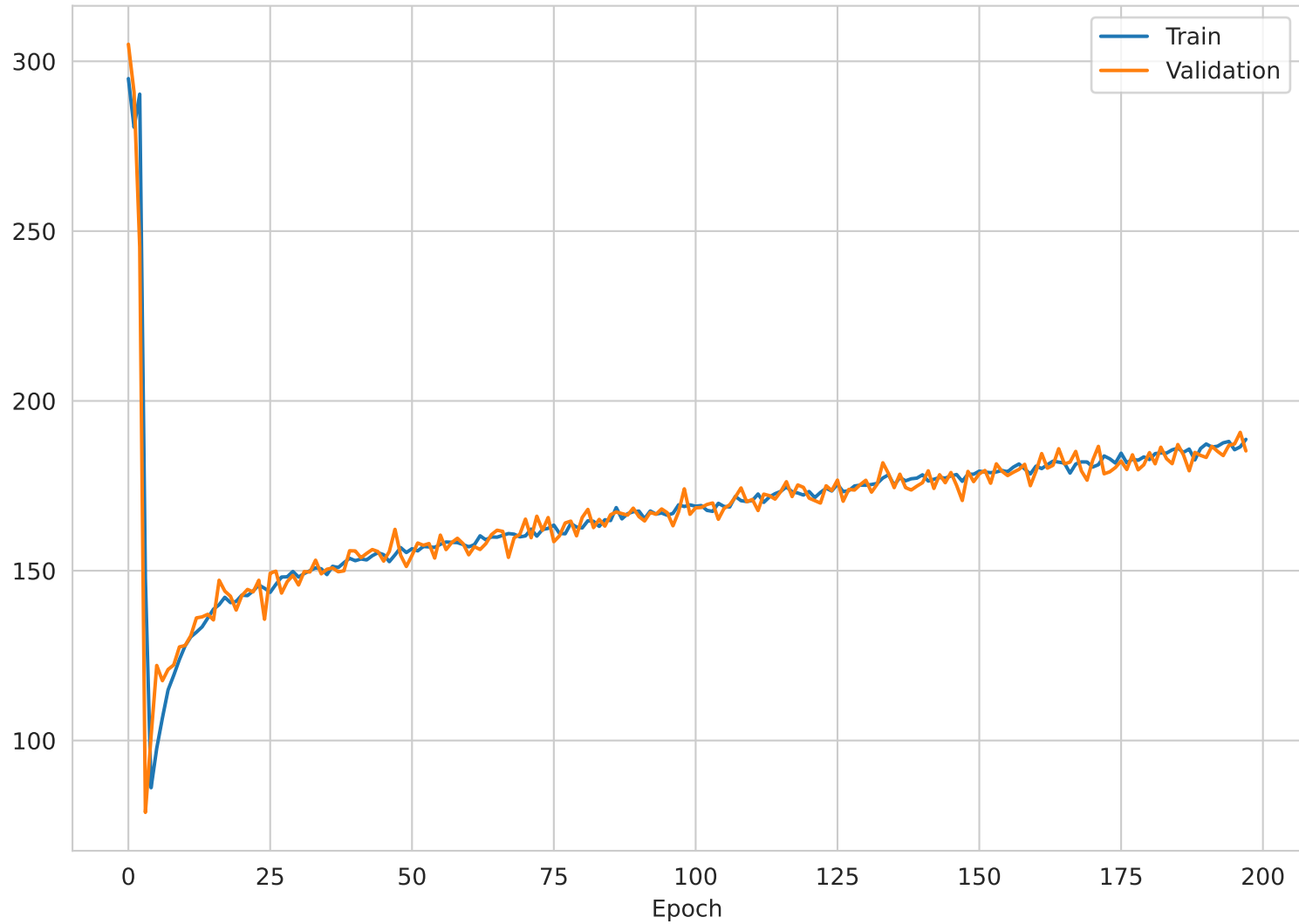
KL Divergence
