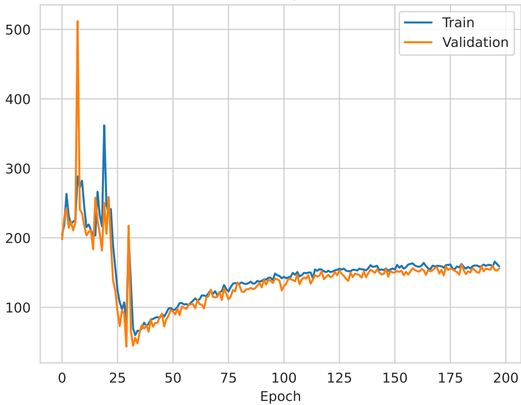
KL Divergence
