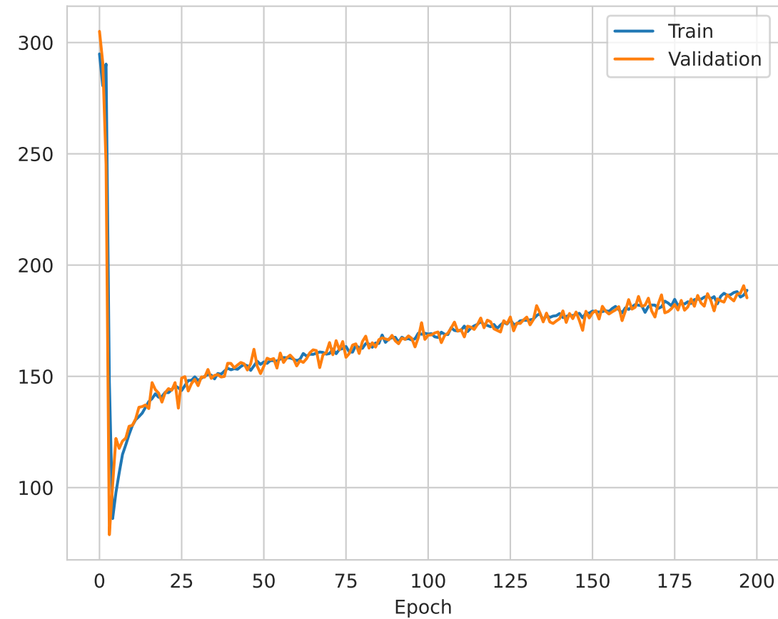
KL Divergence
