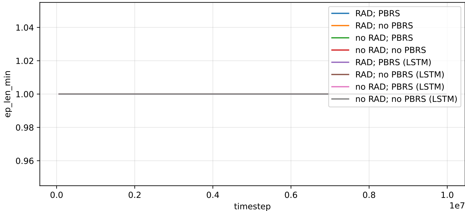
2rooms_2agents -- ep_len_min
