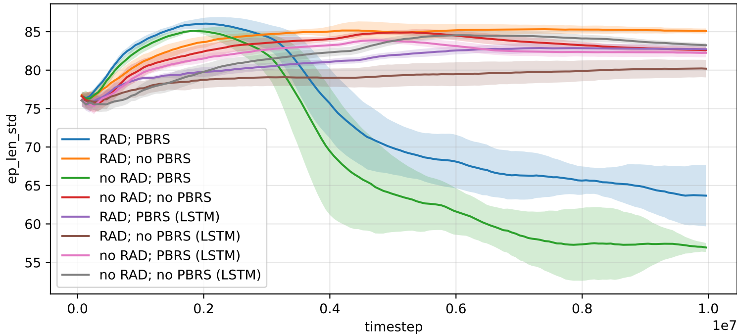
2rooms_2agents -- ep_len_std
