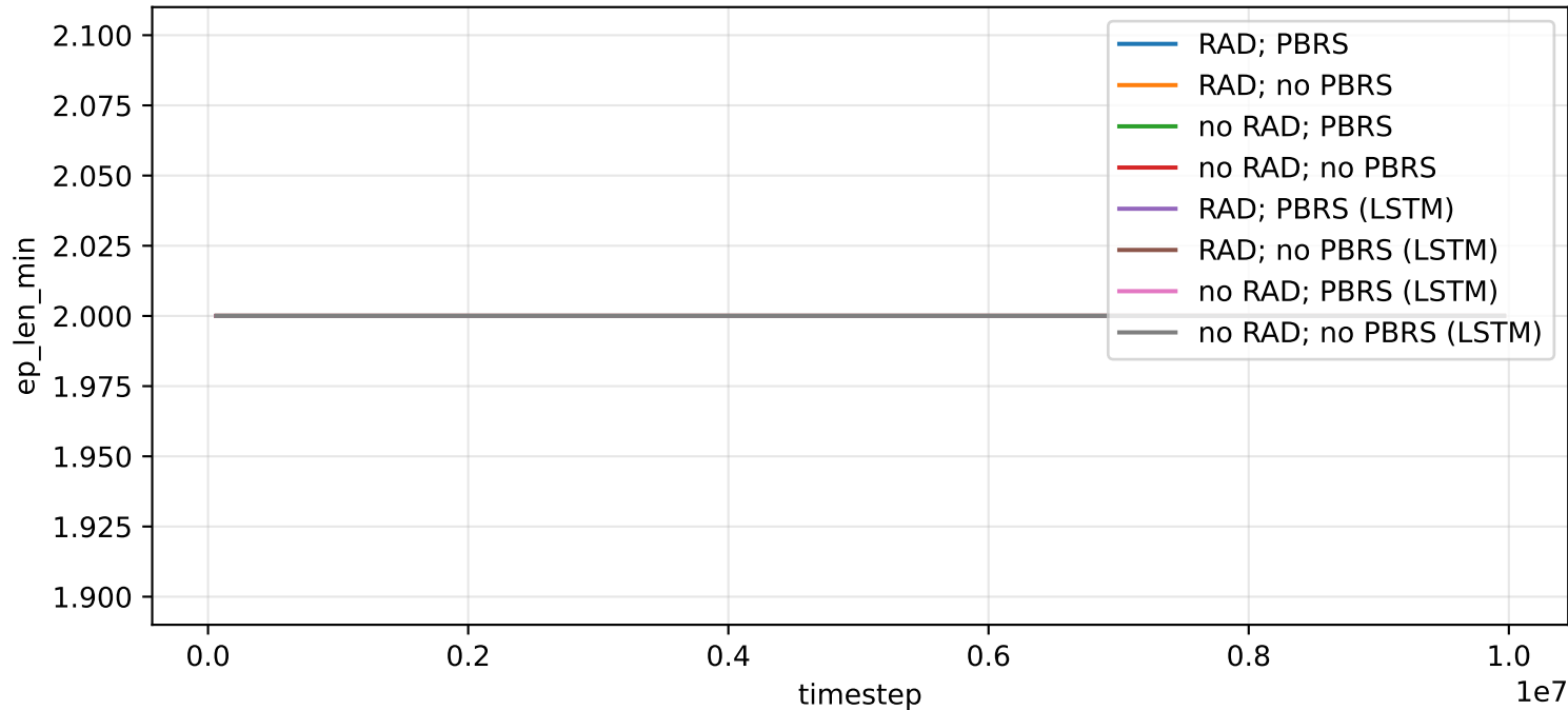
2buttons_2agents -- ep_len_min
