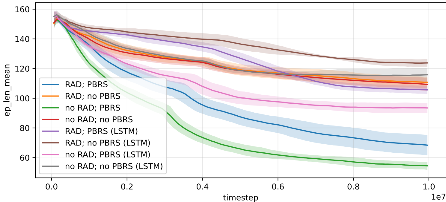
2buttons_2agents -- ep_len_mean
