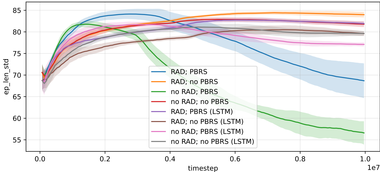
2buttons_2agents -- ep_len_std
