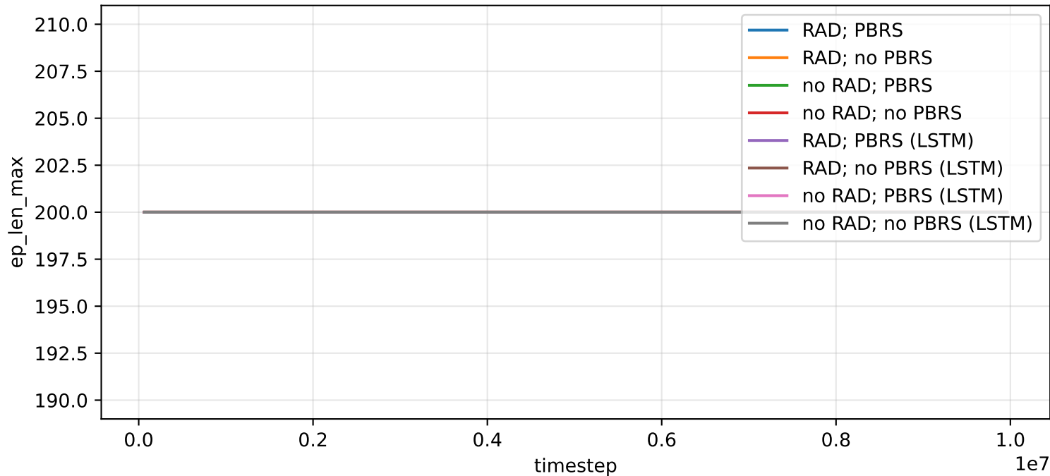
2buttons_2agents -- ep_len_max
