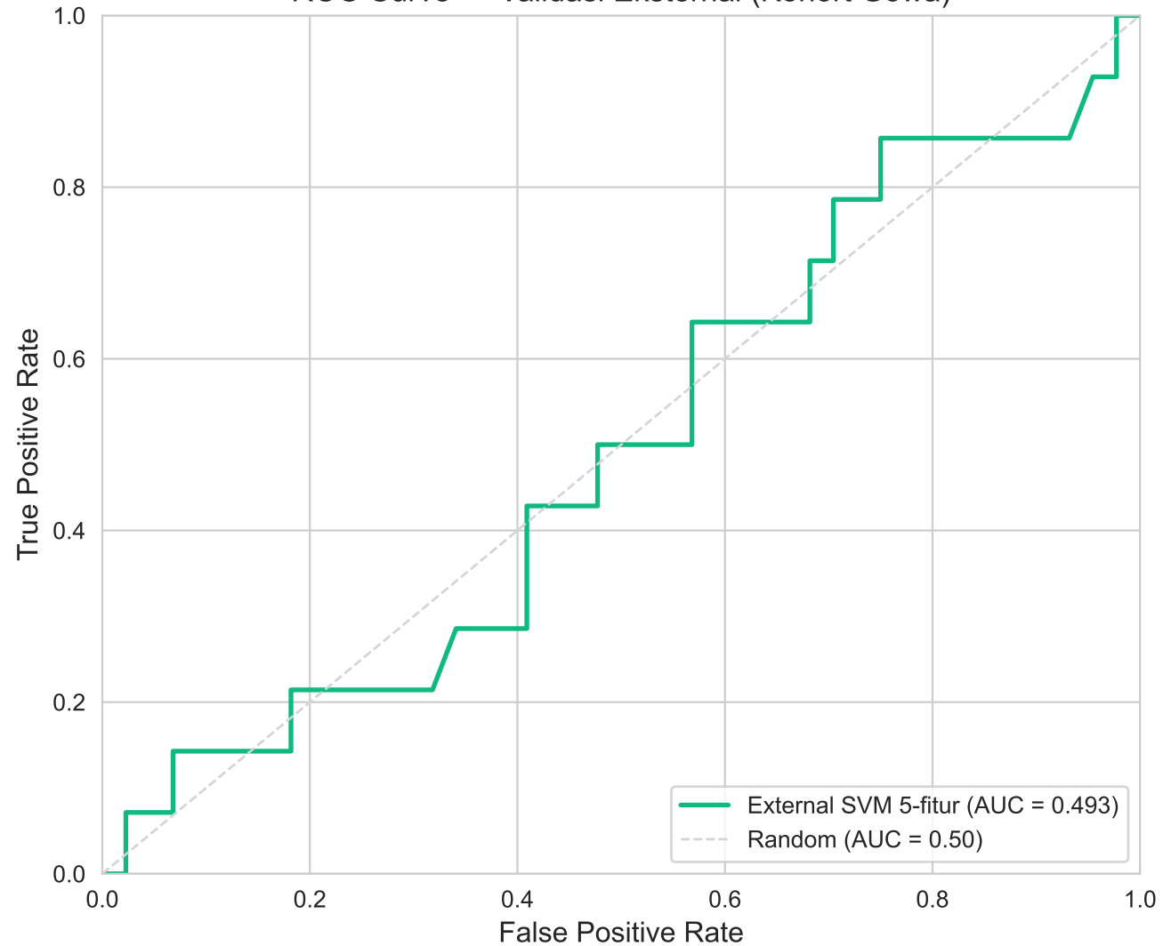
ROC Curve — Validasi Eksternal (Kohort Gowa)
