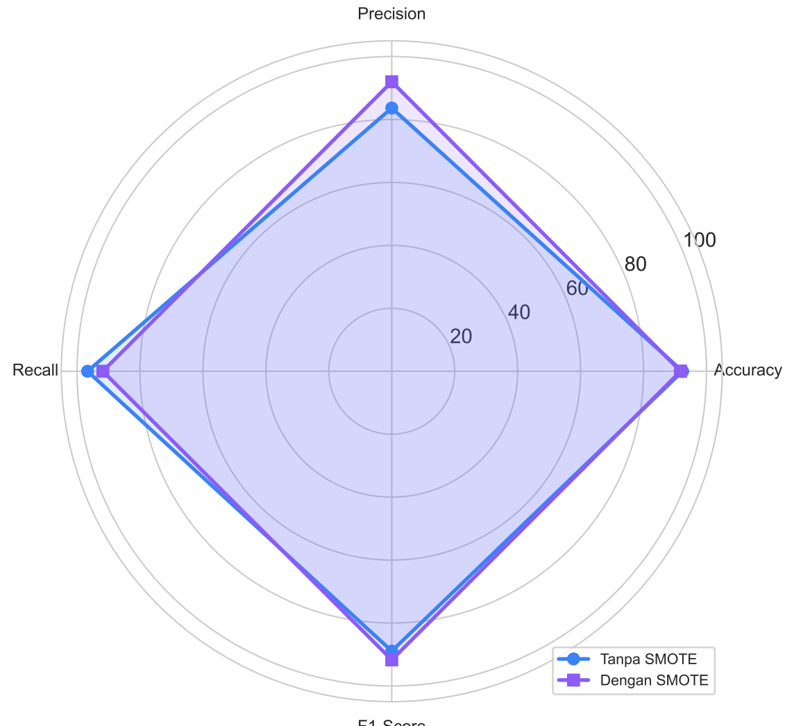
SVM
