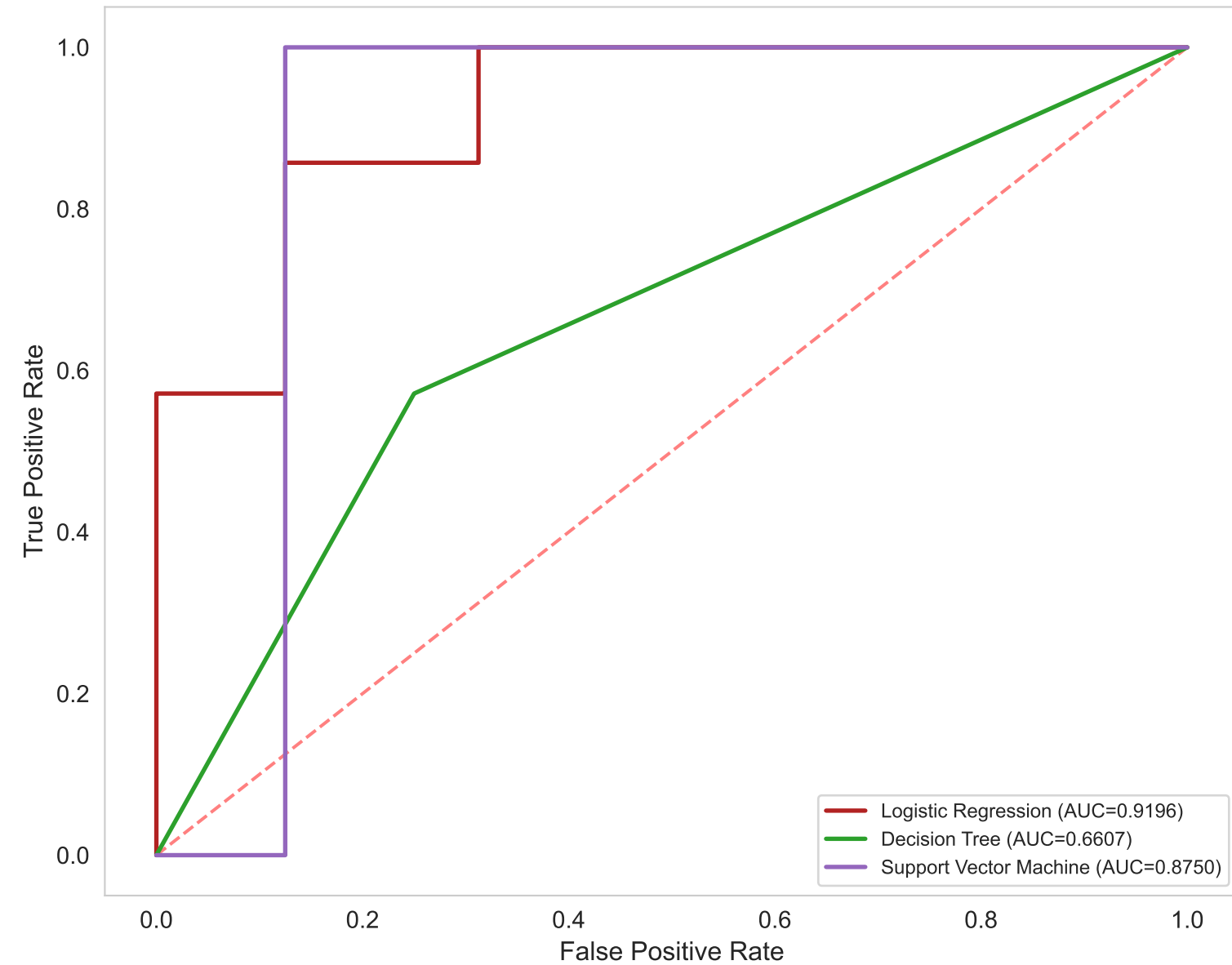
ROC Curve — Dengan SMOTE
