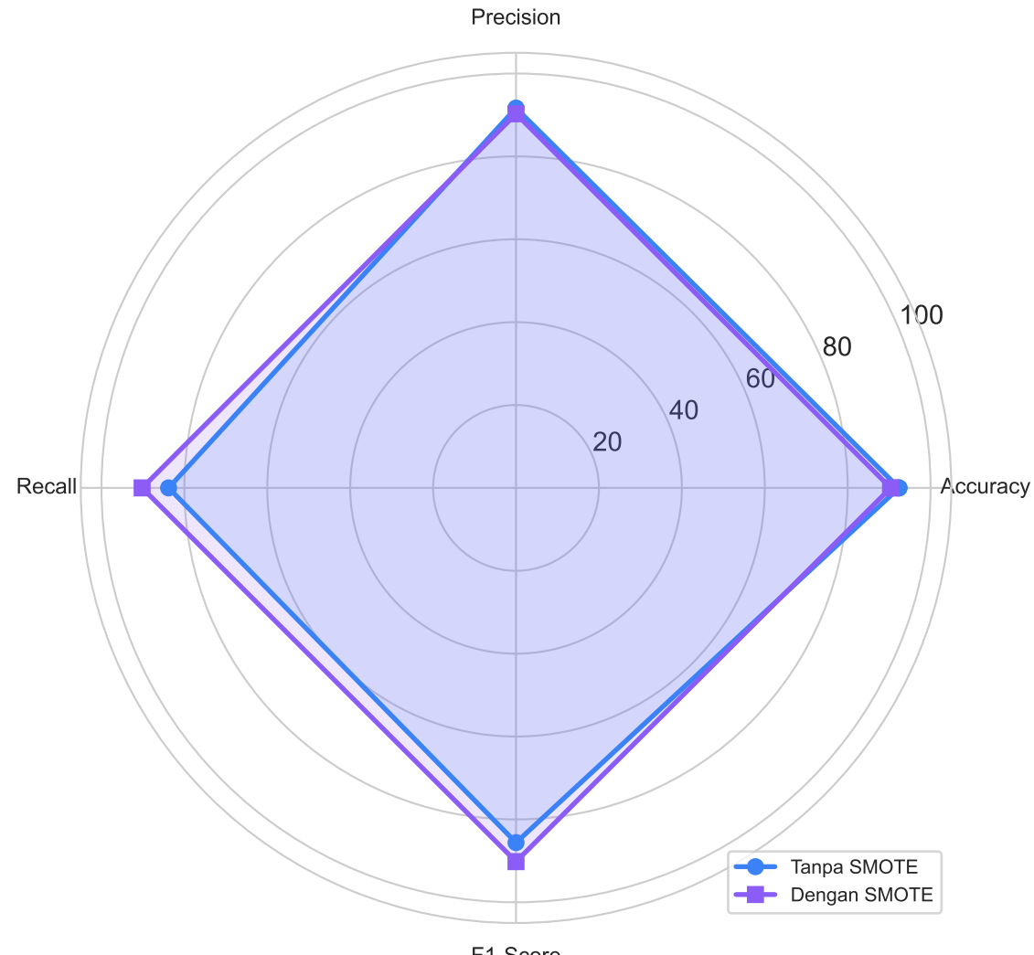
SVM
