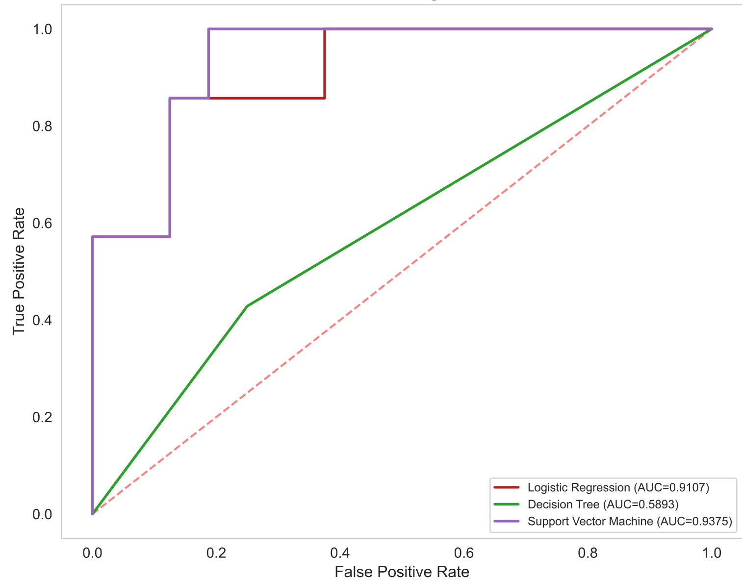
ROC Curve — Dengan SMOTE
