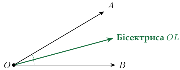
Рис. 11. Бісектриса кута
