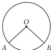
Рис. 14. Центральний кут
