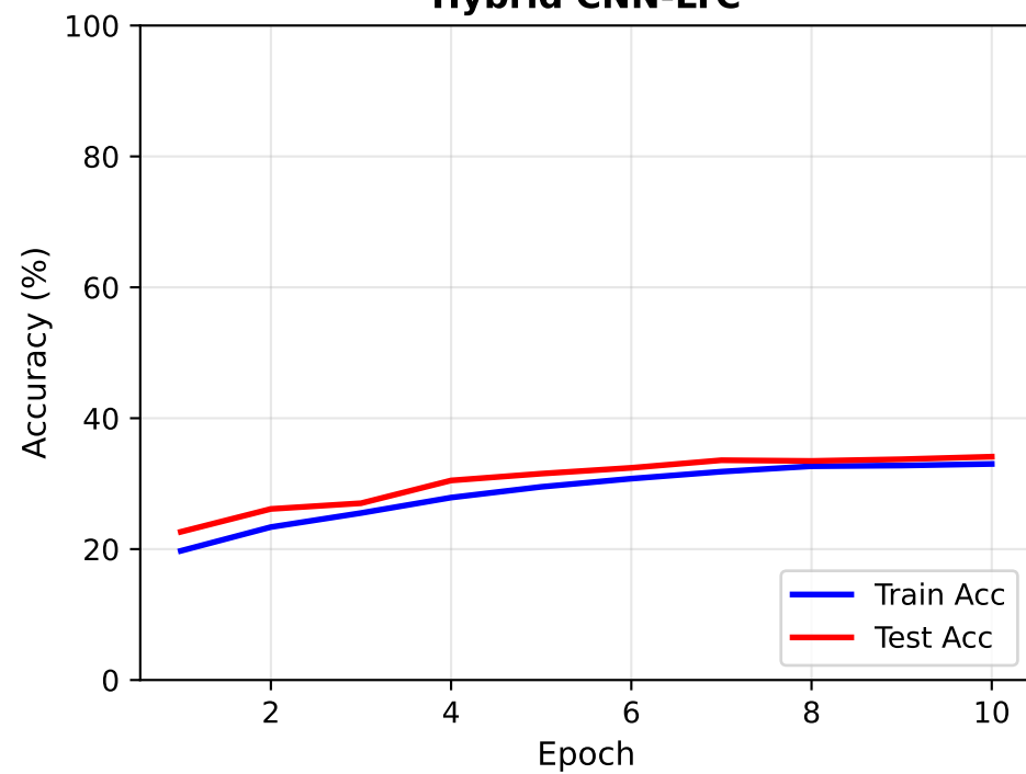
Hybrid CNN-LTC
