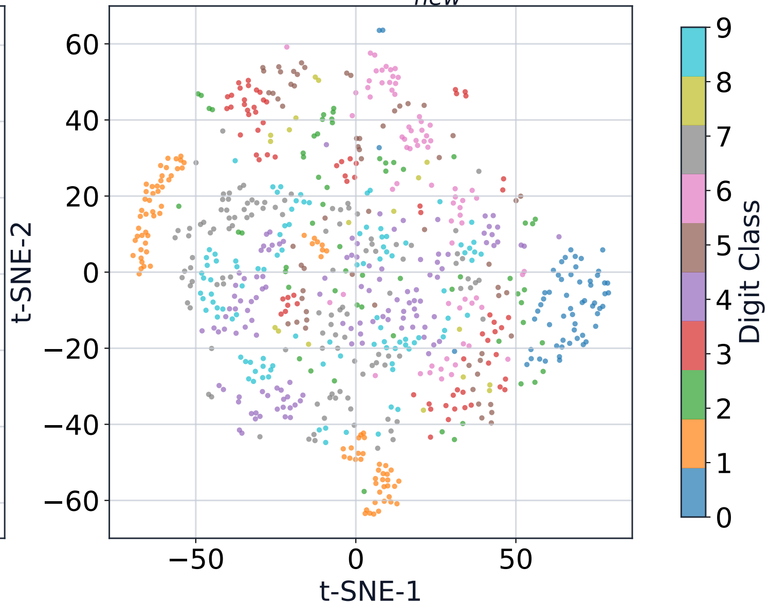
t-SNE: B_{new}^*
