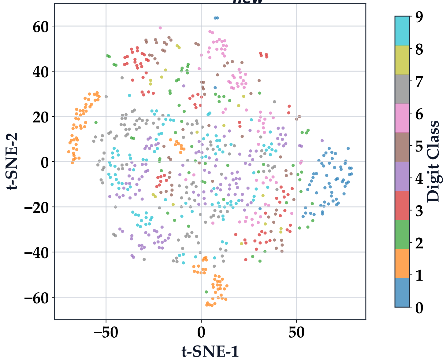
t-SNE: \mathbf{B}_{new}^*
