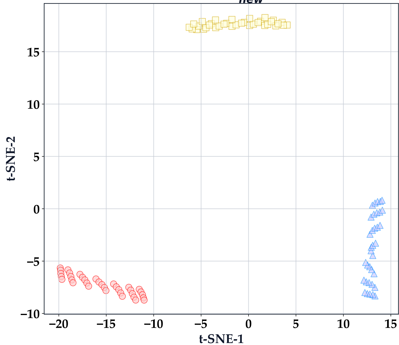
t-SNE: B_{new}^*
