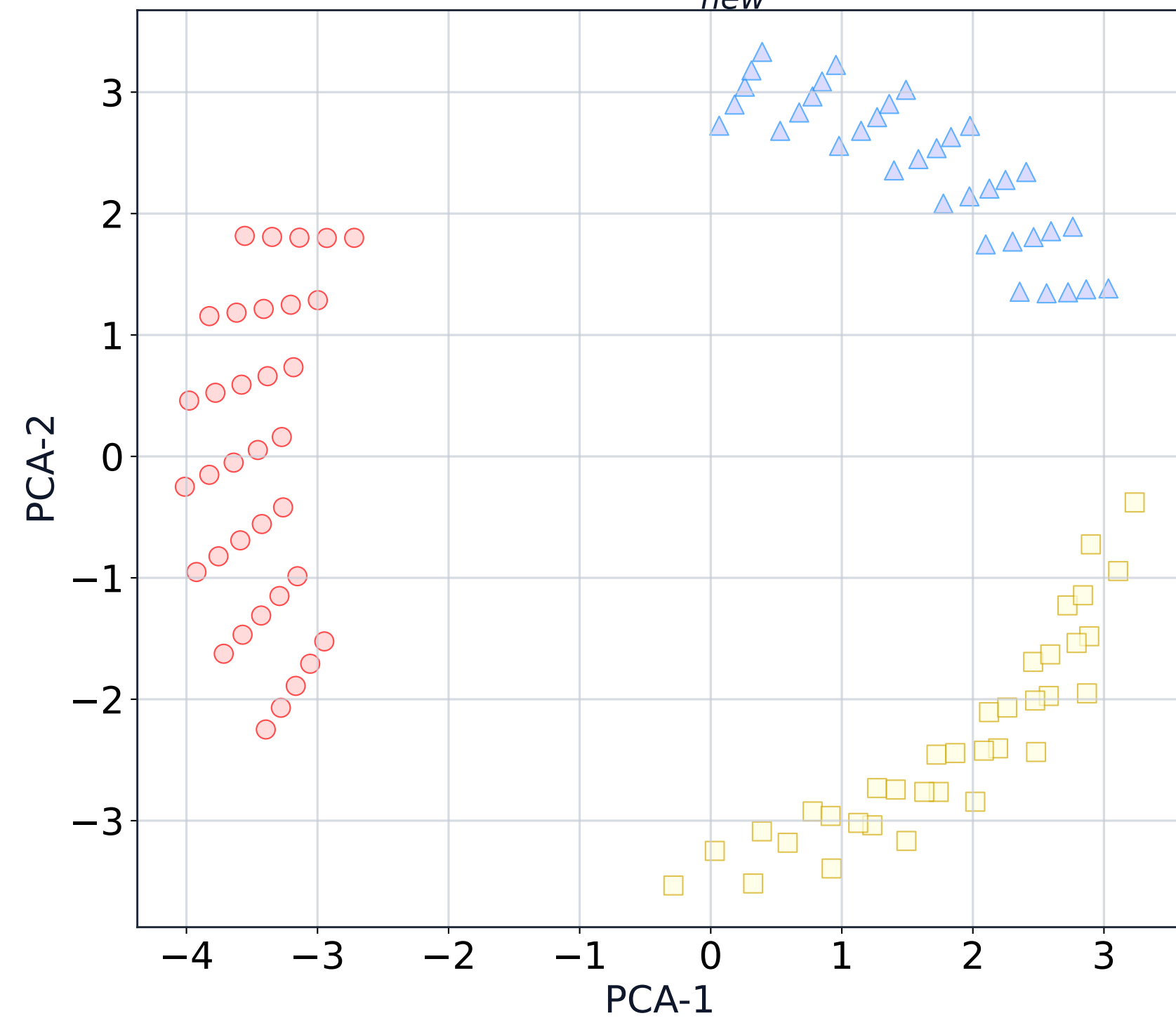
PCA: B_{new}^*
