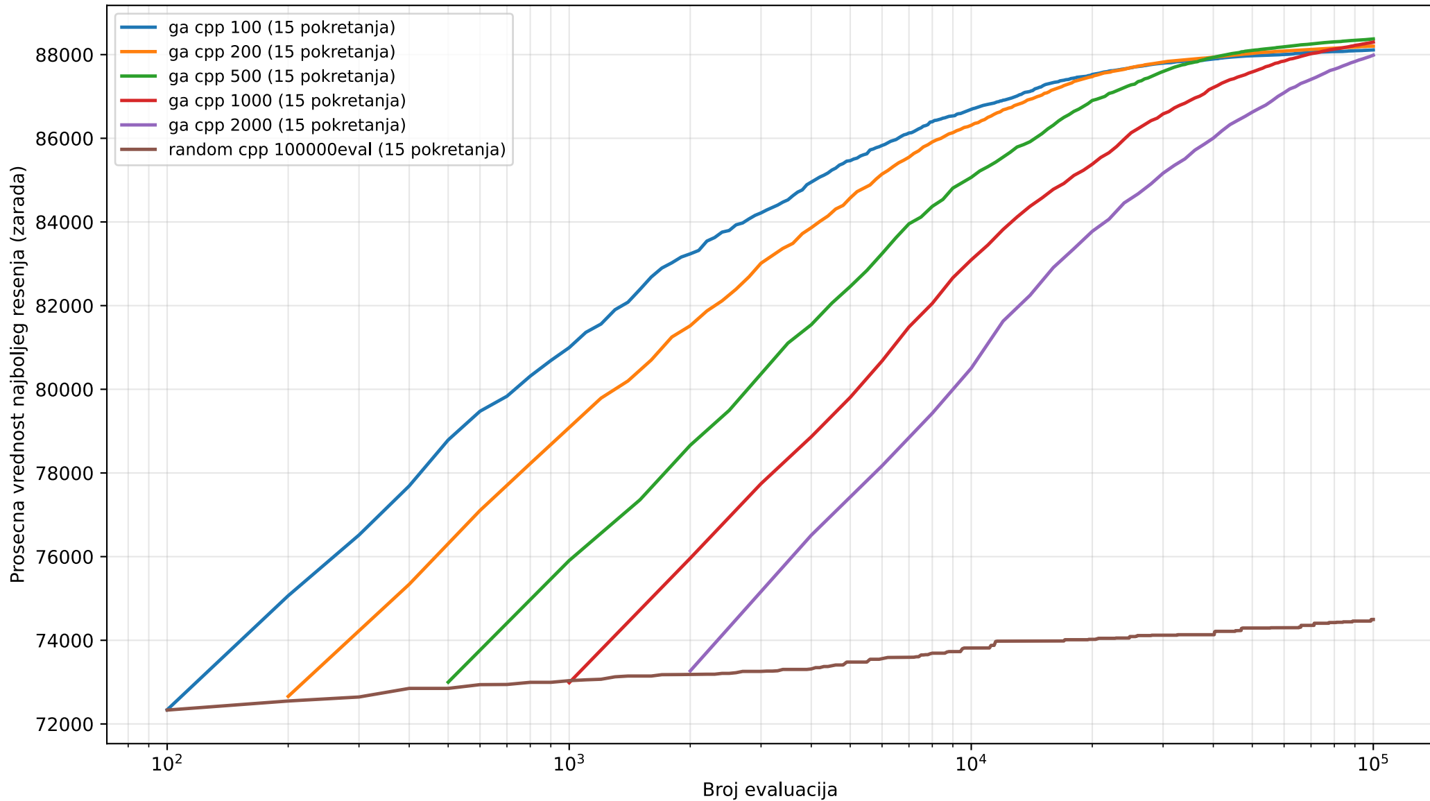
Poredjenje algoritama — prosek po pokretanjima
