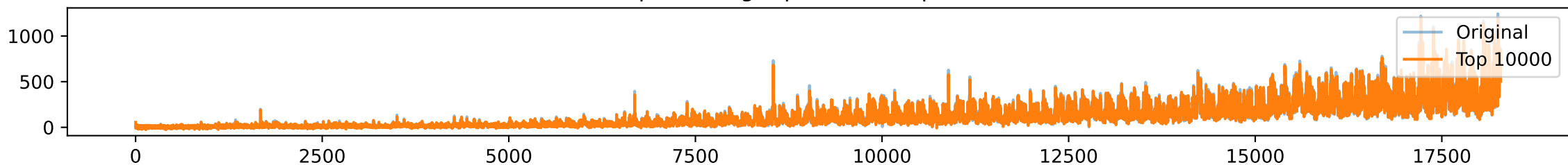
Aprox using top 10000 frequencies
