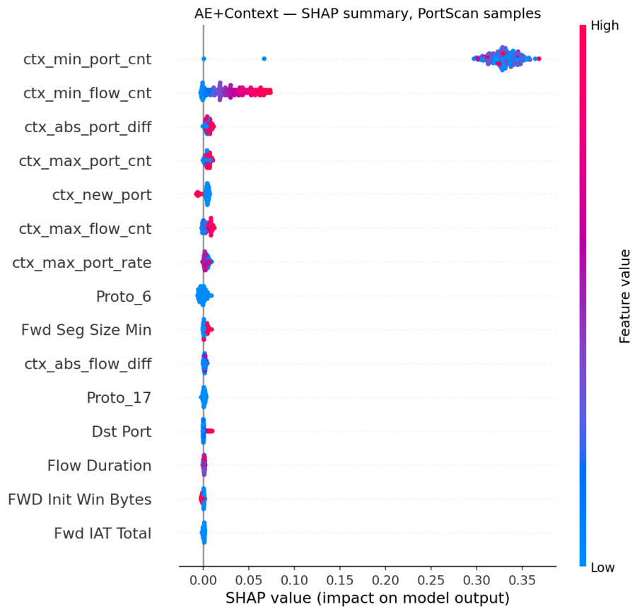
Figura 5.7: AE+Context — diagramă sumară SHAP, eșantioane PortScan. ctx_min_port_cnt domină printr-un cluster strâns, uniform pozitiv, bine separat de orice altă caracteristică; rândurile de top rămase sunt aproape în întregime caracteristici de context al gazdei.
