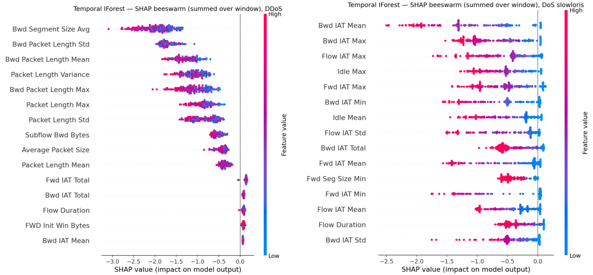
Figura 5.6: Temporal IForest – diagramă beeswarm SHAP per caracteristică, ferestre DDoS (stânga) și ferestre DoS slowloris (dreapta), colapsând axa celor 16 pași temporali prin sumarea contribuției SHAP a fiecărei caracteristici pe toată fereastră și colorând după valoarea medie a acelei caracteristici pe fereastră. DoS slowloris arată o relație monotonă clară – valori mari ale timpului între sosiri (inter-arrival time) determină un SHAP puternic negativ (anormal), valorile mici împing spre zero – consistent cu comportamentul lent, de menținere a conexiunii, după care este numit atacul. DDoS arată o relație valoare-semn mai zgomotoasă pentru caracteristicile sale de lungime a pachetelor pe direcția inversă, și o răspândire per fereastră mai largă decât sugerează, singură, imaginea de medii din Figura 5.4.
