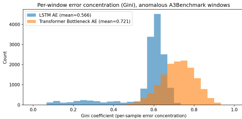
Figura 5.3: Distribuția coeficienților Gini per fereastră, pe toate cele 14,449 ferestre A3 anormale. Distribuția Transformer-ului este unimodală și deplasată spre concentrare ridicată (Gini > 0.6 ); distribuția LSTM Autoencoder-ului este bimodală, cu o majoritate grupată aproape de intervalul Transformer-ului, dar cu o populație secundară distinctă răspândită la valori Gini scăzute.
