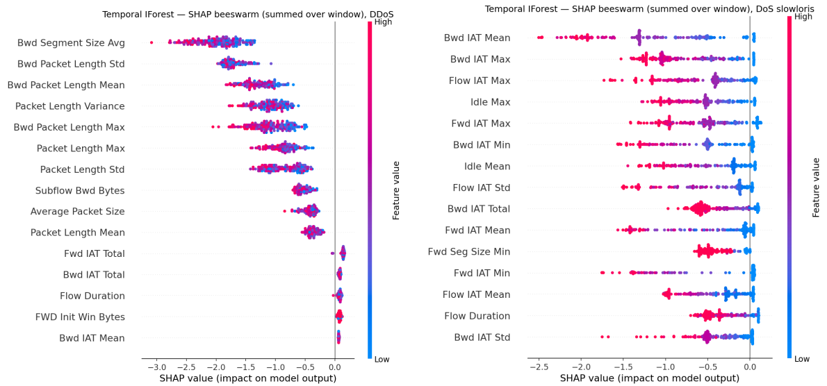
Figura 6.2: Temporal IForest – diagramă beeswarm SHAP per caracteristică, ferestre DDoS (stânga) și ferestre DoS slowloris (dreapta), colapsând axa celor 16 pași temporali prin sumarea contribuției SHAP a fiecărei caracteristici pe toată fereastră și colorând după valoarea medie a acelei caracteristici pe fereastră. DoS slowloris arată o relație monotonă clară – valori mari ale timpului între sosiri (inter-arrival time) determină un SHAP puternic negativ (anormal), valorile mici împing spre zero – consistent cu comportamentul lent, de menținere a conexiunii, după care este numit atacul. DDoS arată o relație valoare-semn mai zgomotoasă pentru caracteristicile sale de lungime a pachetelor pe direcția inversă, și o răspândire per fereastră mai largă decât sugerează, singură, imaginea de medii din Figura 5.4.
