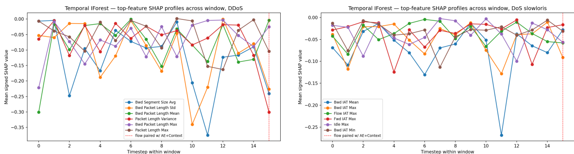
Figura 5.4: Temporal IForest – valoarea medie SHAP per pas temporal pentru cele șase caracteristici cu cea mai mare atribuire, ferestre DDoS (stânga) și ferestre DoS slowloris (dreapta). În ambele cazuri atribuirea este negativă (anormală), recurentă cu semn consistent pe majoritatea celor 16 pași temporali, și nu se concentrează pe fluxul final (linia roșie punctată) – fluxul combinat cu scorul lui AE+Context în ansamblul propus.
