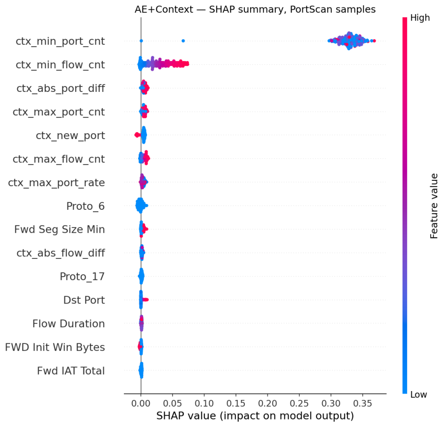
Figura 5.5: AE+Context – diagramă sumară SHAP, eșantioane PortScan. ctx_min_port_cnt domină printr-un cluster strâns, uniform pozitiv, bine separat de orice altă caracteristică; rândurile de top rămase sunt aproape în întregime caracteristici de context al gazdei.
