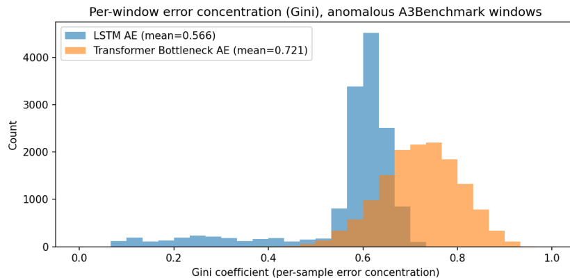
Figura 5.3: Distribuția coeficienților Gini per fereastră, pe toate cele 14,449 ferestre A3 anormale. Distribuția Transformer-ului este unimodală și deplasată spre concentrare ridicată (Gini > 0.6); distribuția LSTM Autoencoder-ului este bimodală, cu o majoritate grupată aproape de intervalul Transformer-ului, dar cu o populație secundară distinctă răspândită la valori Gini scăzute.
