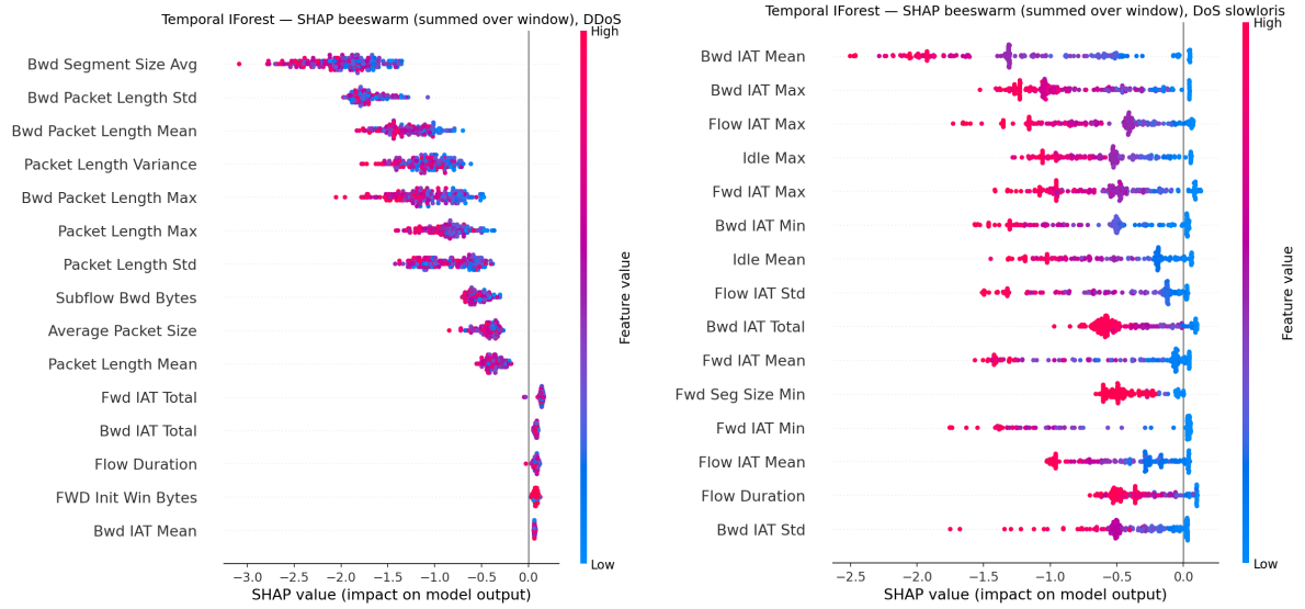
Figura 5.2: Temporal IForest – diagramă beeswarm SHAP per caracteristică, ferestre DDoS (stânga) și ferestre DoS slowloris (dreapta), colapsând axa celor 16 pași temporali prin sumarea contribuției SHAP a fiecărei caracteristici pe toată fereastră și colorând după valoarea medie a acelei caracteristici pe fereastră. DoS slowloris arată o relație monotonă clară – valori mari ale timpului între sosiri (inter-arrival time) determină un SHAP puternic negativ (anormal), valorile mici împing spre zero – consistent cu comportamentul lent, de menținere a conexiunii, după care este numit atacul. DDoS arată o relație valoare-semn mai zgomotoasă pentru caracteristicile sale de lungime a pachetelor pe direcția inversă, și o răspândire per fereastră mai largă decât sugerează, singură, imaginea de medii din Figura 5.4.
