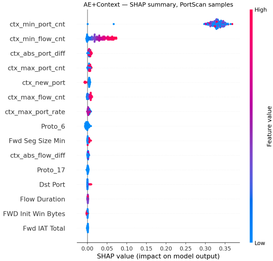
Figura 5.7: AE+Context – diagramă sumară SHAP, eşantioane PortScan. ctx_min_port_cnt domină printr-un cluster strâns, uniform pozitiv, bine separat de orice altă caracteristică; rândurile de top rămase sunt aproape în întregime caracteristici de context al gazdei.
