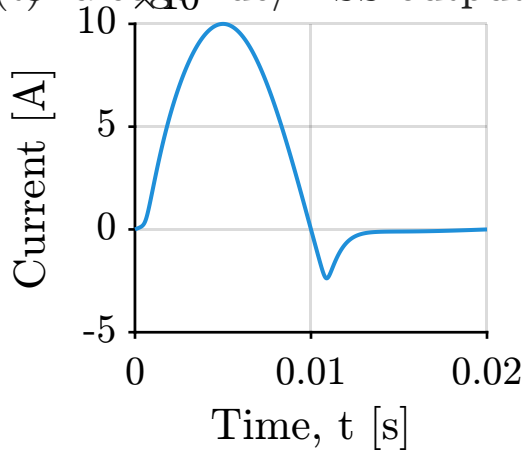
Chalcogenide/MSS output i(t)
