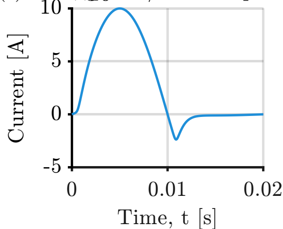
Chalcogenide/MSS output i(t)
