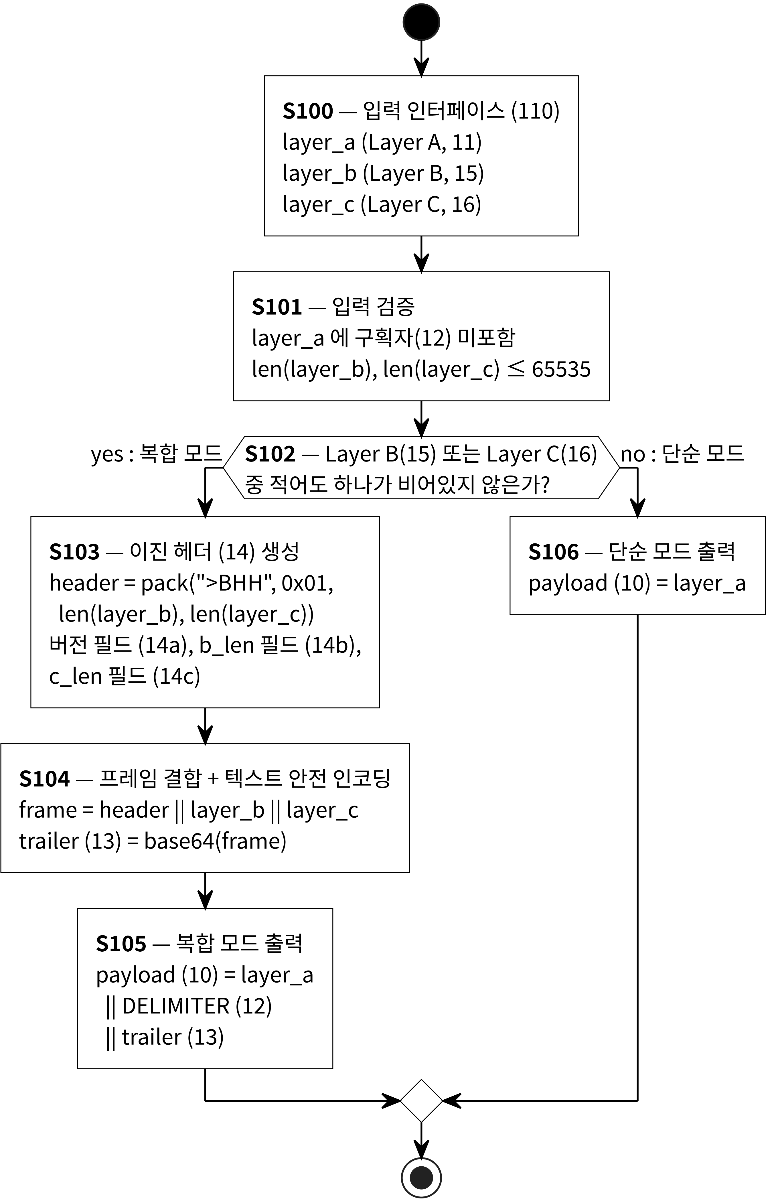
Fig. 2 — 인코더 (130) 의 동작 흐름
